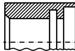
Рисунок 4.10 – Размеры проточки
