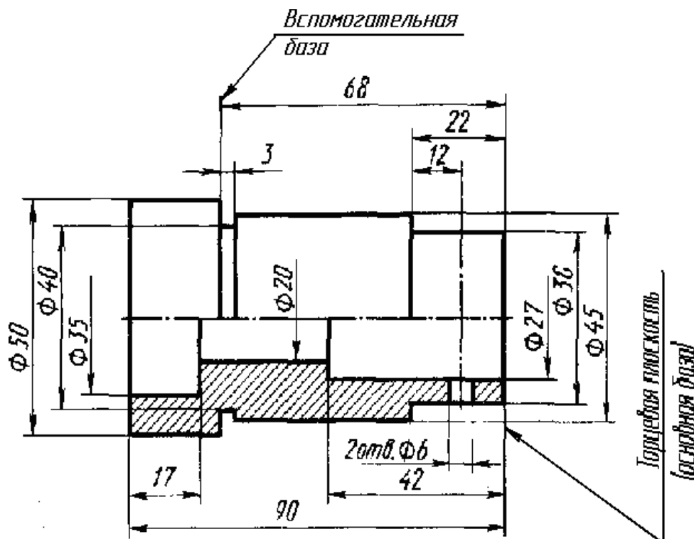
Рисунок 4.28 – Вспомогательная база
