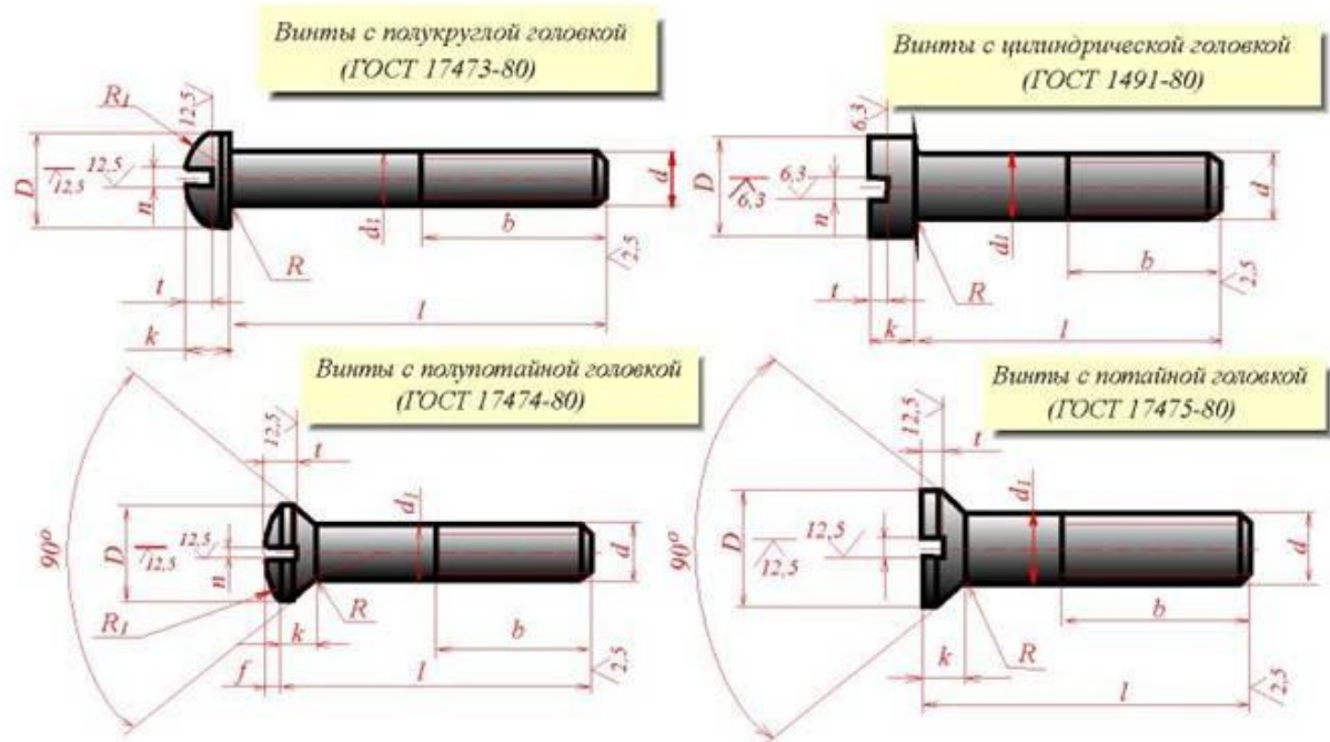
Рисунок 3.18 – Винт
