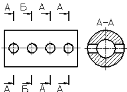
Рисунок 2.26 – Оформление нескольких одинаковых сечений.
