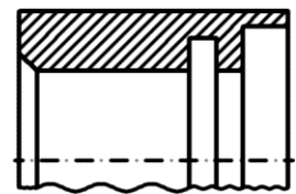
Рисунок 4.10 – Размеры проточки
