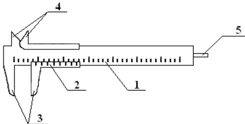
Рисунок 2.3 – Штангенциркуль
