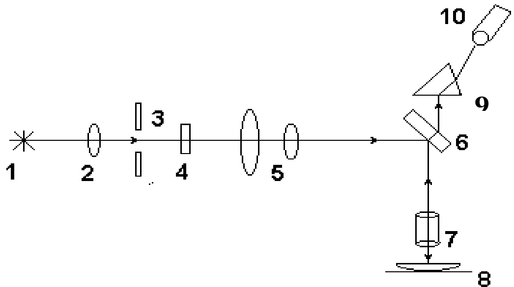
Рисунок 20.4 – Принципиальная схема установки
