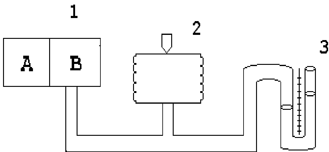
Рисунок 19.3 – Принципиальная схема регулирования и измерения давления: 1 – кюветы; 2 – сильфон с вентилем; 3 – манометр (водяной)
