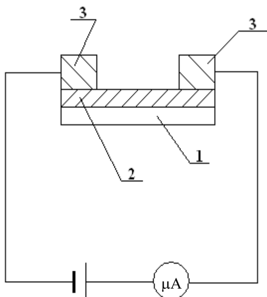
Рисунок 24.2 – Схема фотосопротивления
