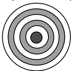
Рисунок 20.2 – Кольца Ньютона
