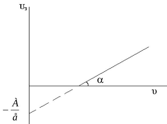
Рисунок 25.3 – Зависимость задерживающего потенциала от частоты света
