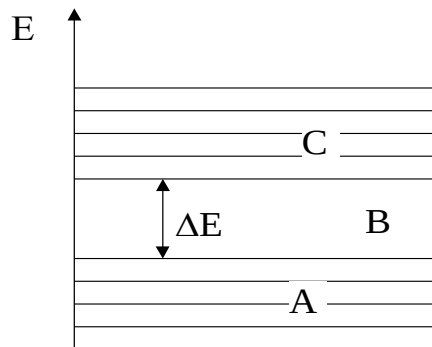
Рисунок 15.1 – Энергетические зоны полупроводника
