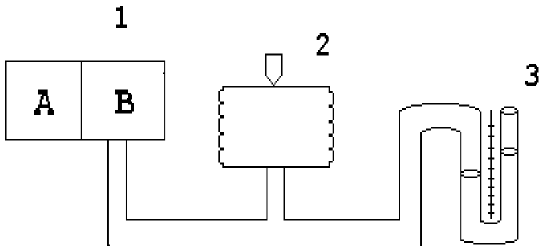
Рисунок 19.2 – Рабочая схема интерферометра ШИ-5
