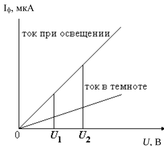
Рисунок 24.3 – Вольт-амперные характеристики \Phi C
