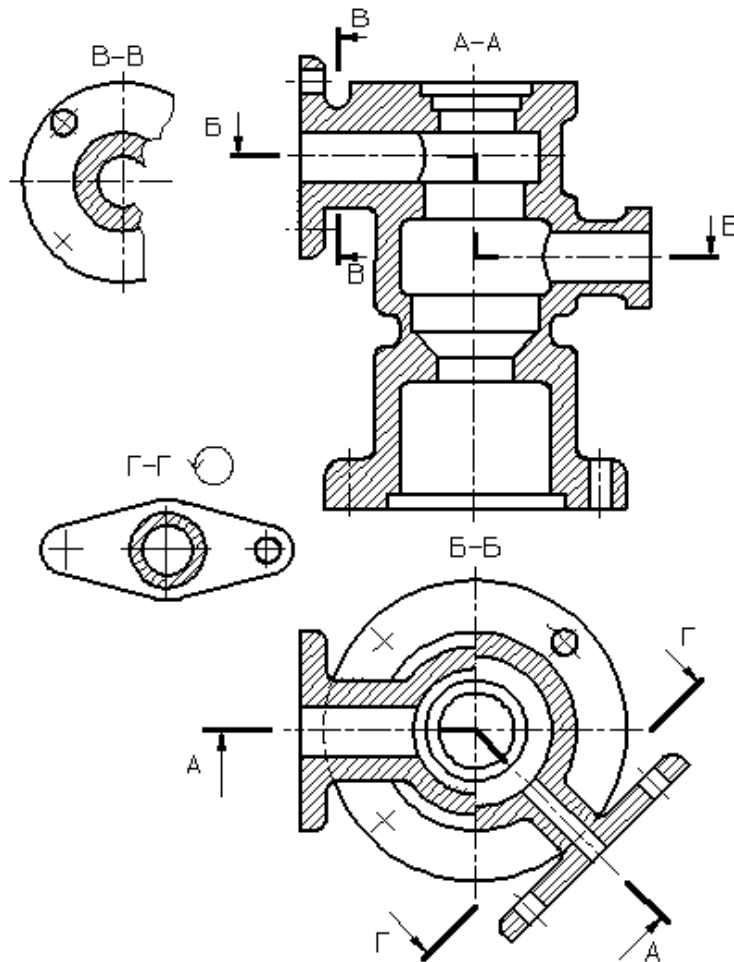
Рисунок 2.7 – Виды разрезов.
