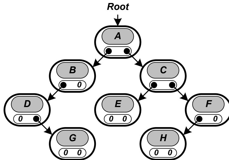
Рисунок 3.4 — Бинарное дерево
