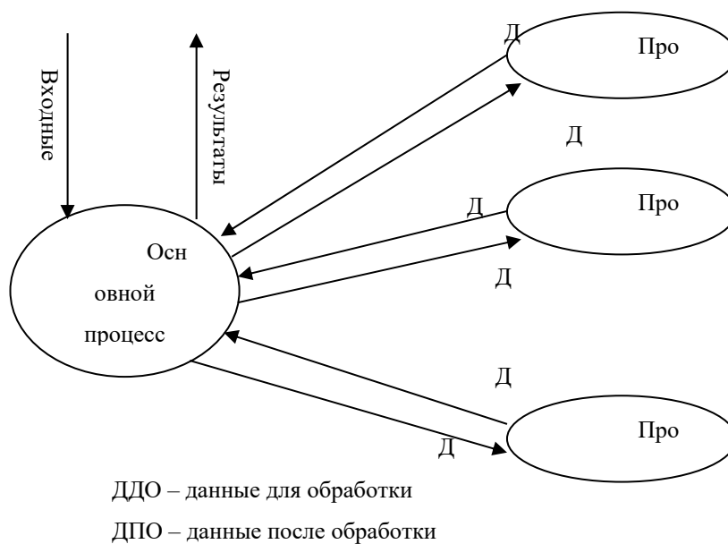
Рис. 1. Схема взаимодействия частей SPMD-программы.
