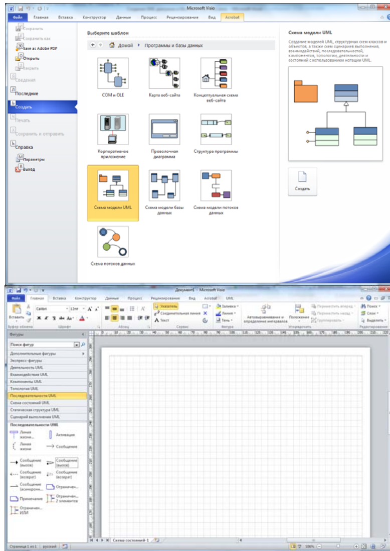
Интерфейс Visio 2010
