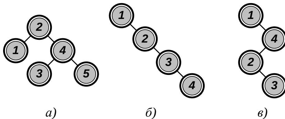
Рисунок 3.12 — Формирование бинарного дерева поиска при включении элементов: а) случайным образом; б) в порядке возрастания; в) сериями монотонности
