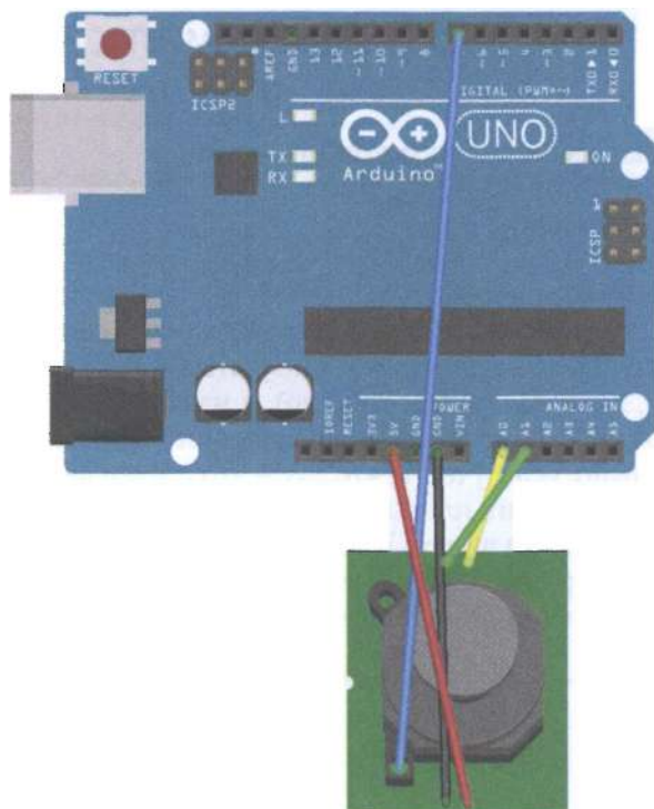
Рис. 104 ❖ Схема подключения для практического занятия 31
