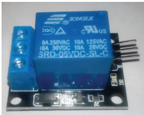
Рис. 25 ❖ Релейный модуль
