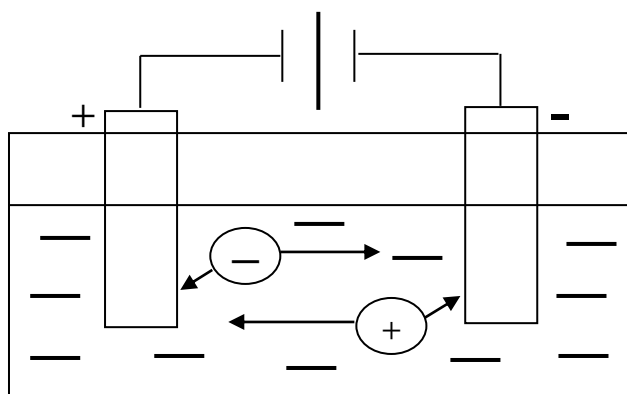
Рисунок 9.1 Схема электролизёра
