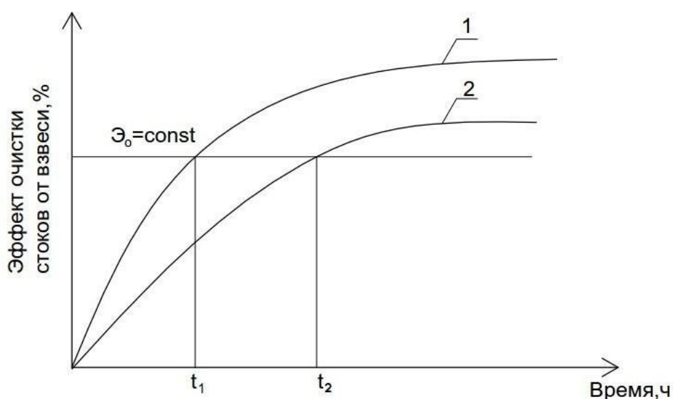
Рис. 9.1. Определение времени отстаивания в цилиндрах: 1 — зависимость \Theta_{в.в.} = f(t) при глубине воды в цилиндре h_1 ; 2 — зависимость \Theta_{в.в.} = f(t) при глубине воды в цилиндре h_2
