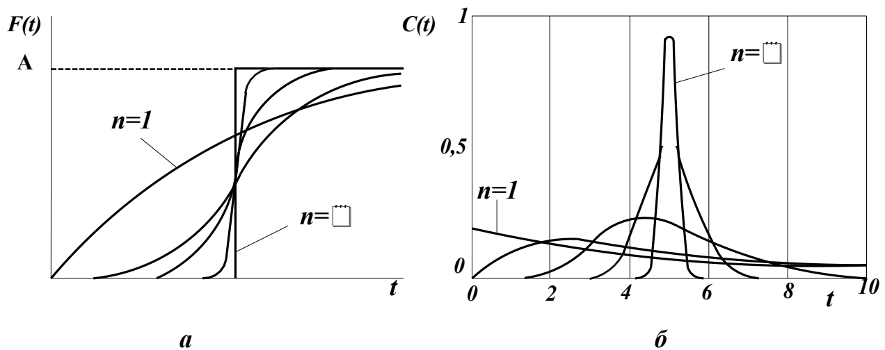
а – F-кривые; б – С-кривые.
