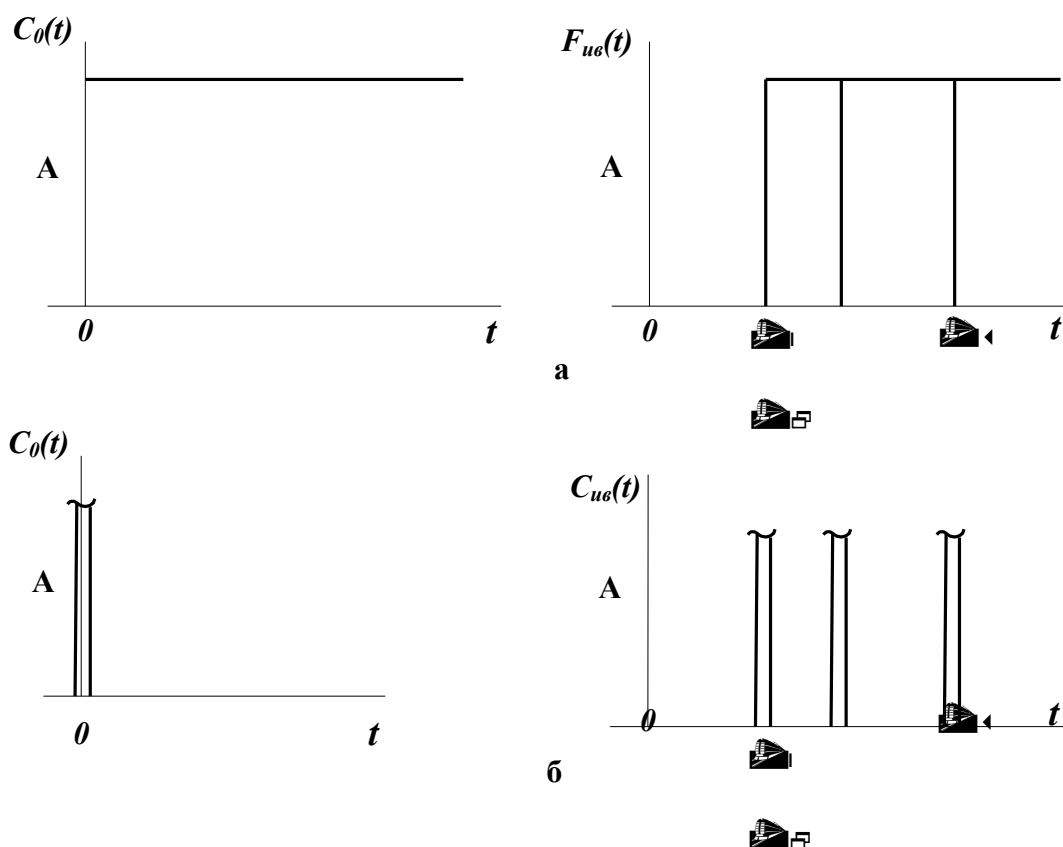
а – F-кривые; б – С-кривые, где t_1, t_2, t_3 – время запаздывания Рисунок 4.4 – Характеристики модели аппарата ИВ
