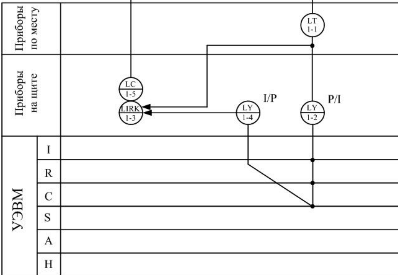
Рисунок 1.1 – Схема автоматизации процесса регулирования уровня воды в резервуаре
