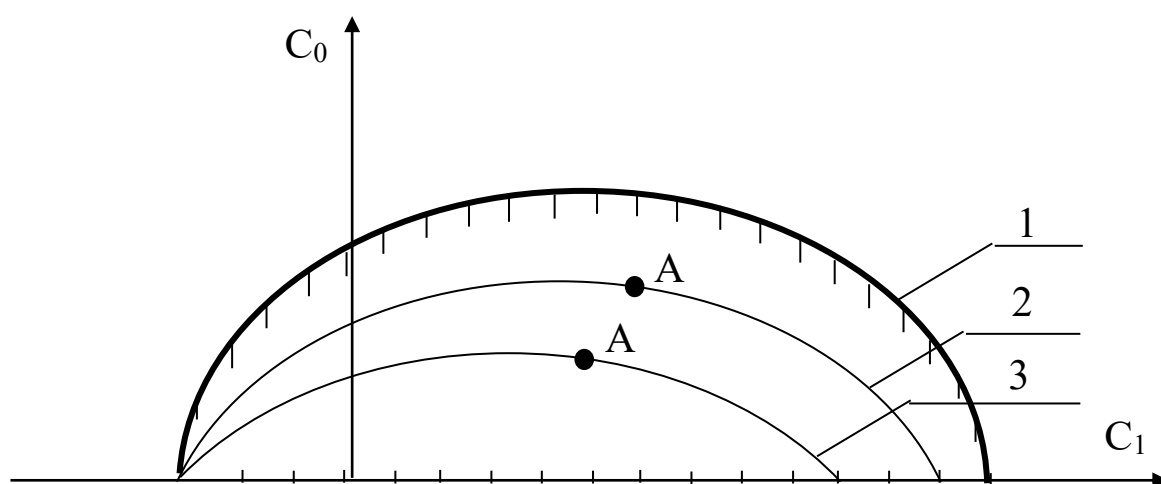
Рисунок 3 – Разбиение области устойчивости в плоскости параметров настройки ПИ-регулятора: 1 – граница области устойчивости ( m = 0 );
