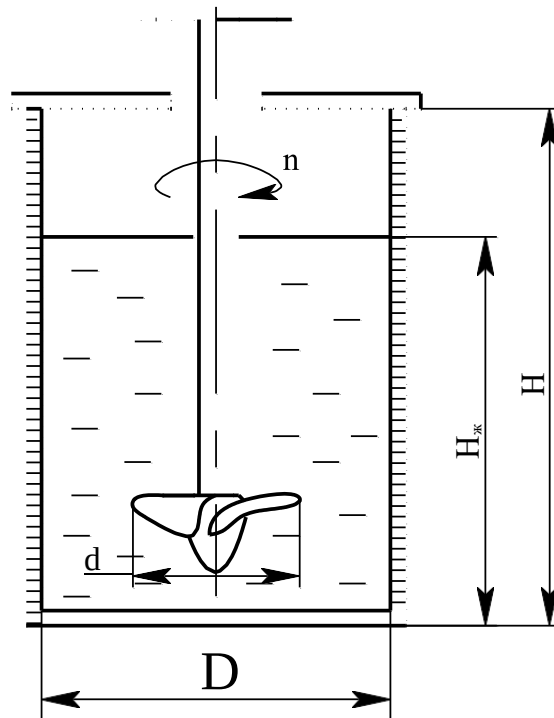
Рисунок 2.8 – Схема к расчету мешалки
