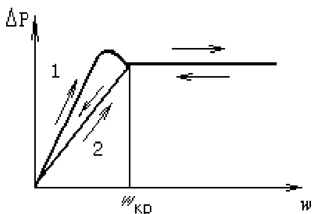
Рисунок 3 Потеря напора в реальном слое: 1 - кривая прямого хода; 2 - кривая обратного хода.
