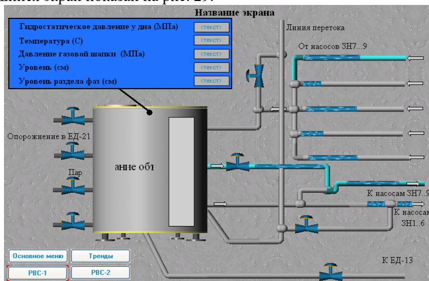
Рис. 29. Экран PBC с размещенными кнопками
