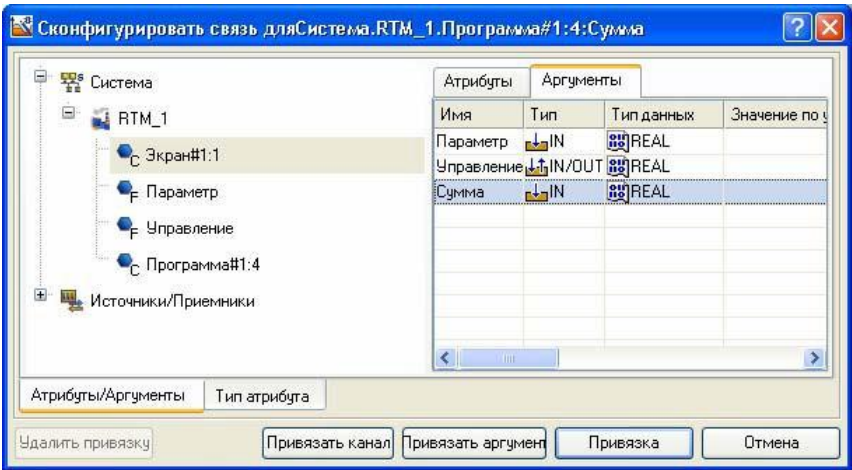
Рисунок 53 – Привязка аргументов программы к атрибутам каналов В результате, будем иметь рисунок 54.
