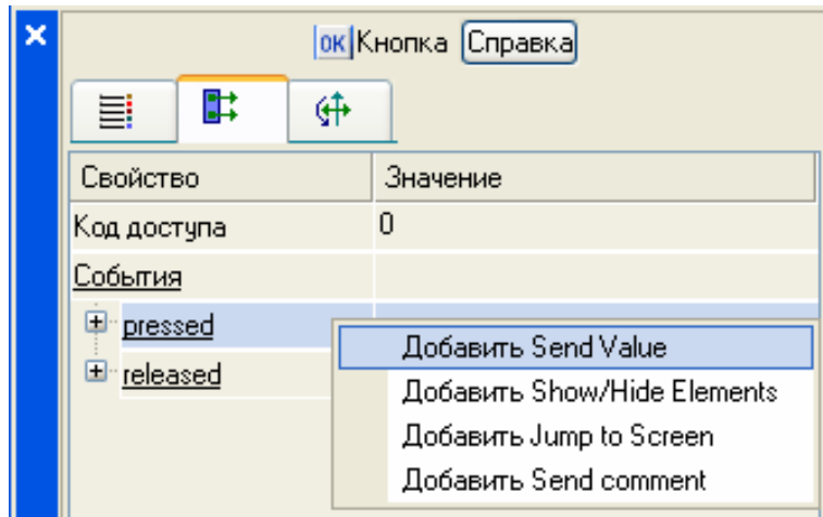
Рисунок 31 – Настройка графического элемента Кнопка
