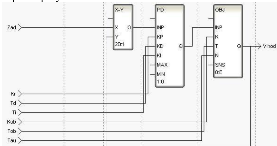
Рисунок 111 – Программа реализации системы управления
