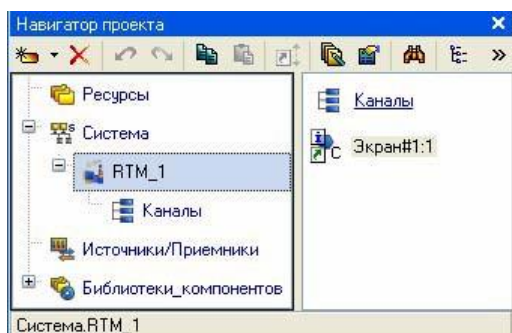
Рисунок 91 – Навигатор проекта
