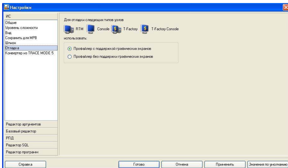
Рисунок 62 – Настройки ИСР
