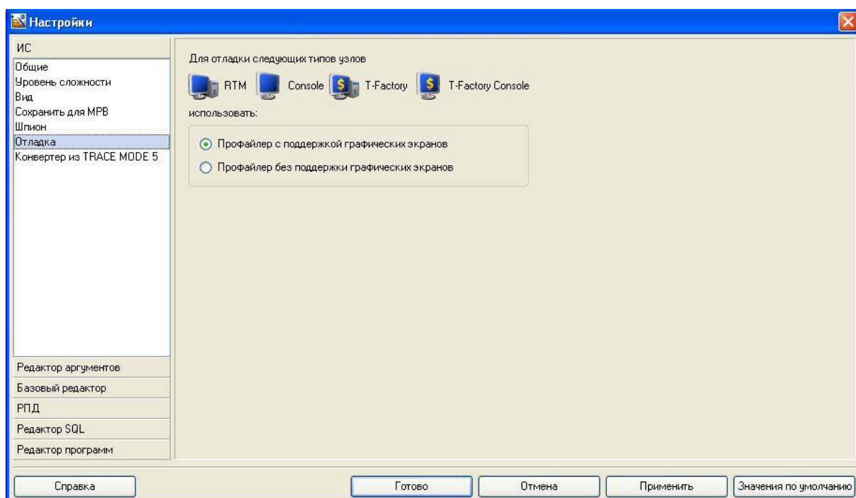
Рисунок 13 – Настройки ИСП
