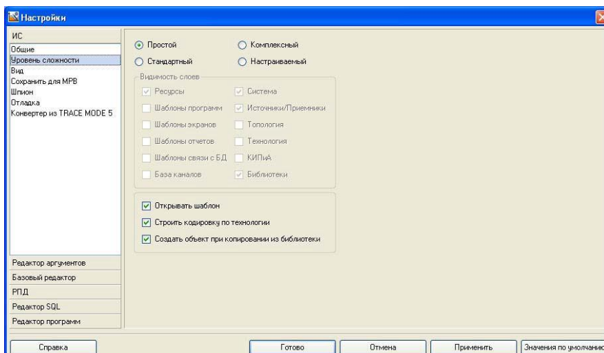
Рисунок 88 – Настройки ИСР
