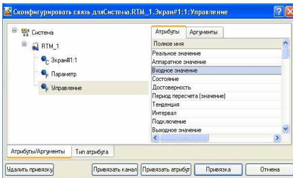
Рисунок 38 – Конфигурация системы Закрывать окно
