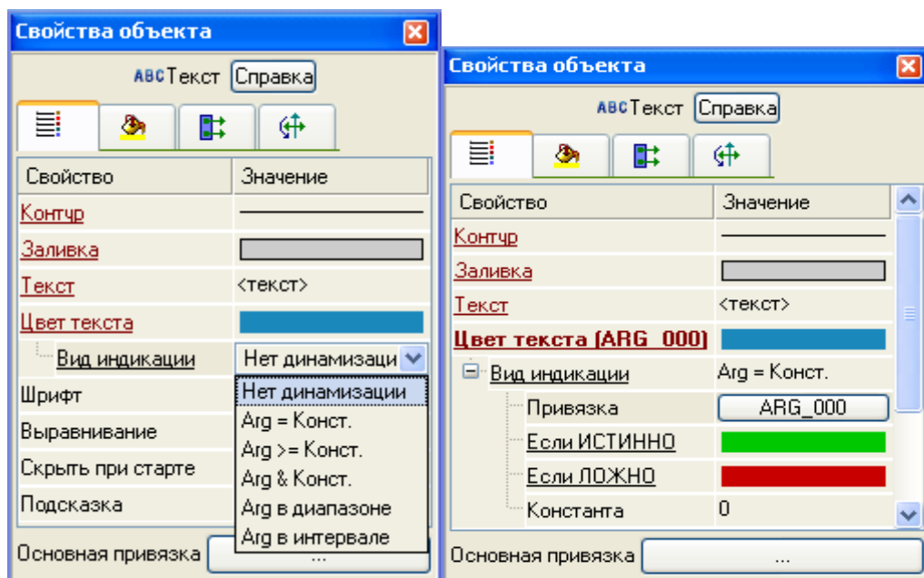
Рис. 26. Динамизация атрибутов
