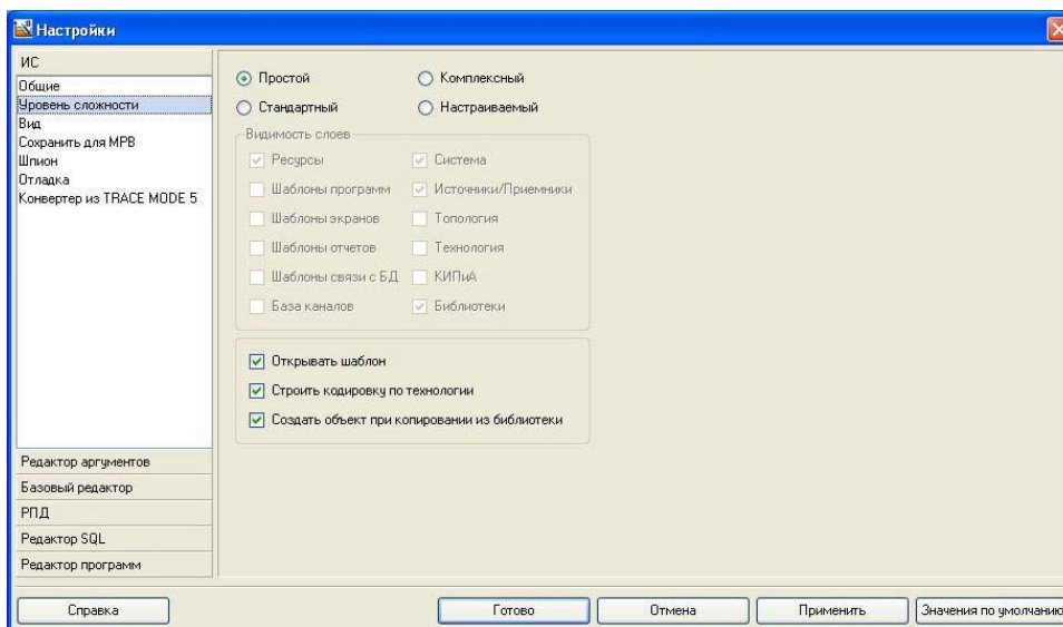
Рисунок 61 – Настройки ИСР
