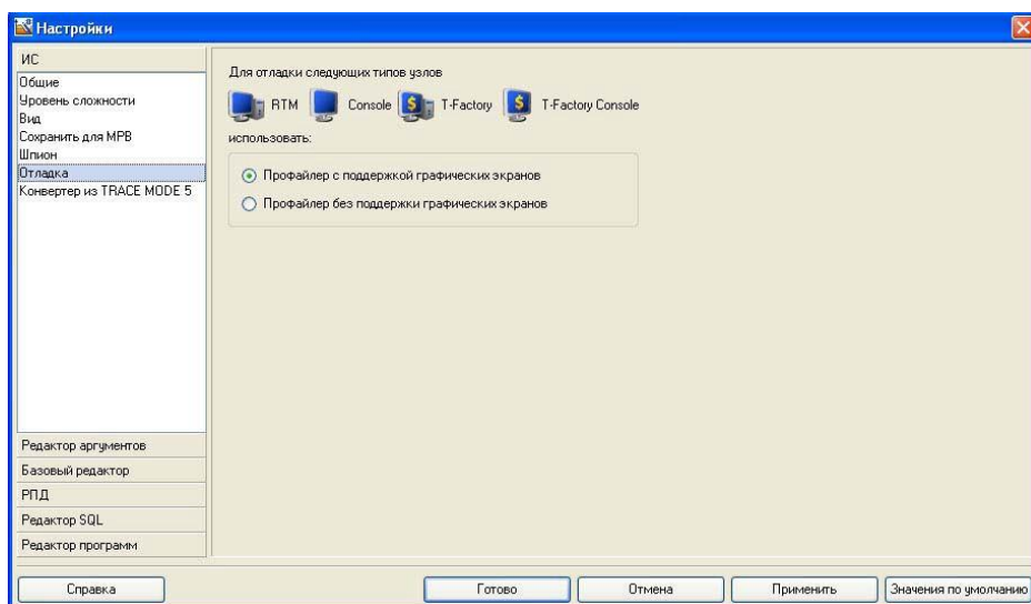
Рисунок 89 – Настройки ИСР
