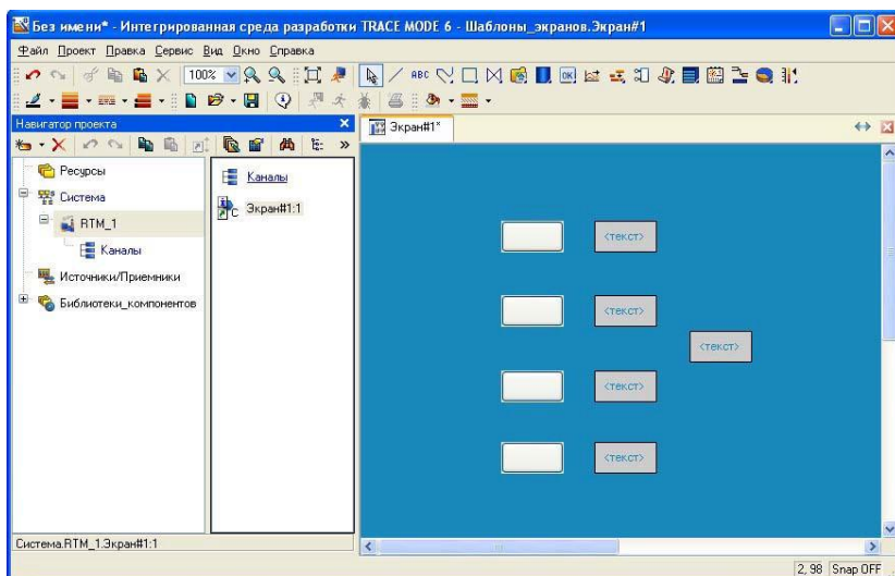
Рисунок 70 – Графический экран
