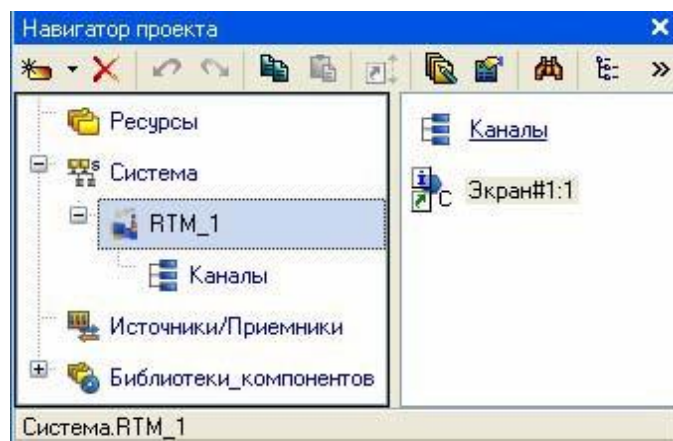
Рисунок 15 – Навигатор проекта
