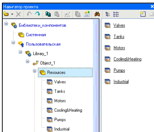
Рис. 5. Навигатор проекта
