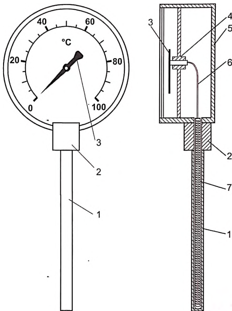
Рис. 2.4. Биметаллический термометр
