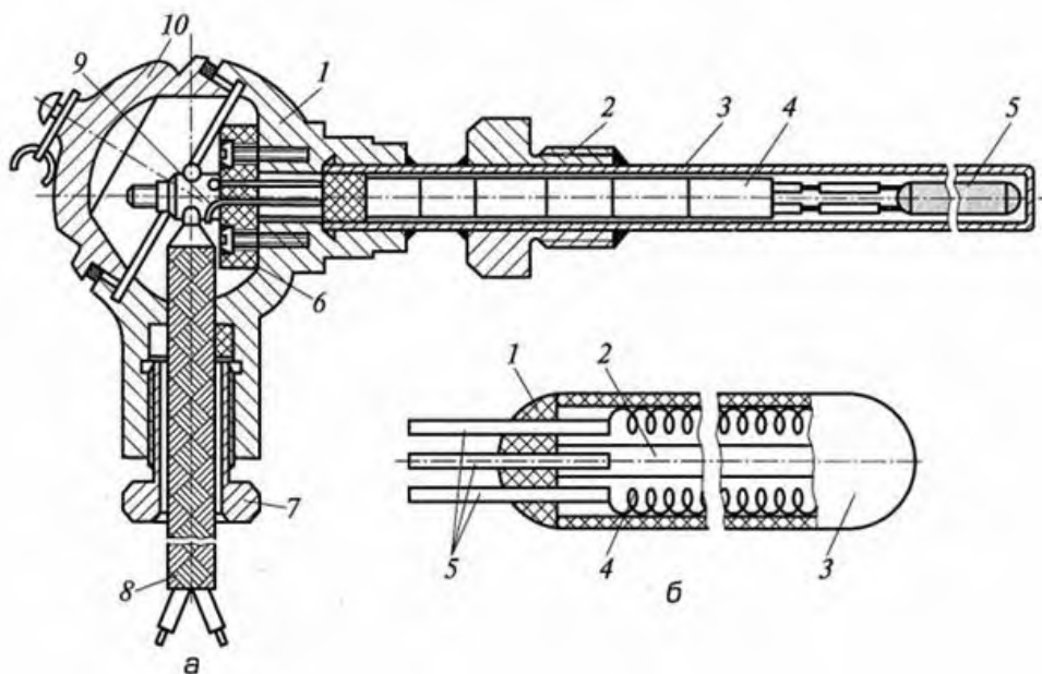
Рис. 2.6. Термометр сопротивления
