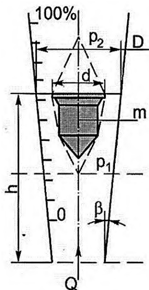
Рис. 6.3. Схема ротаметра
