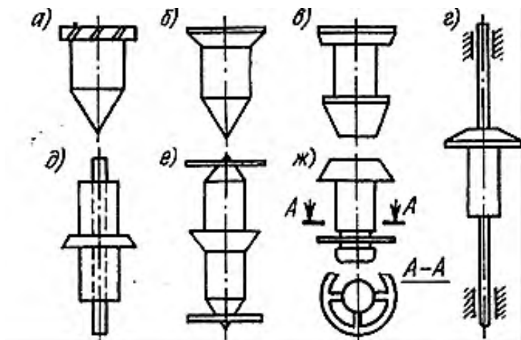
Рис. 6.2. Формы поплавков
