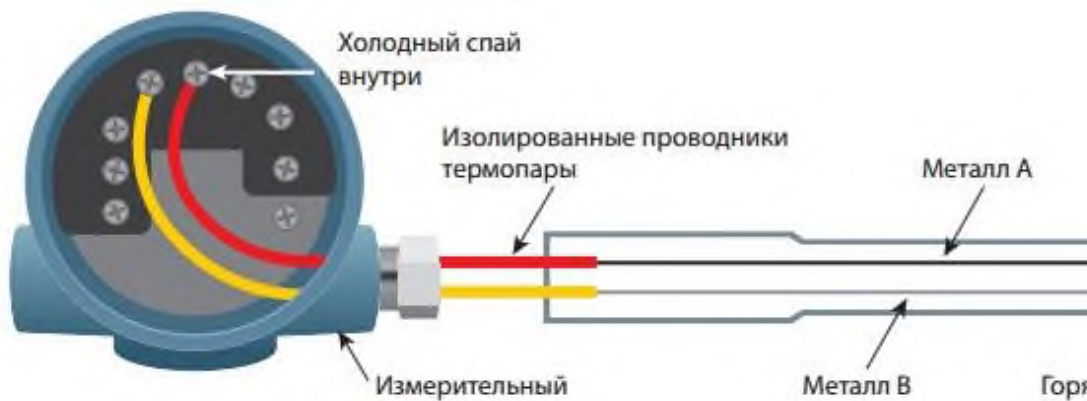
Рисунок 2.5. Термопара
