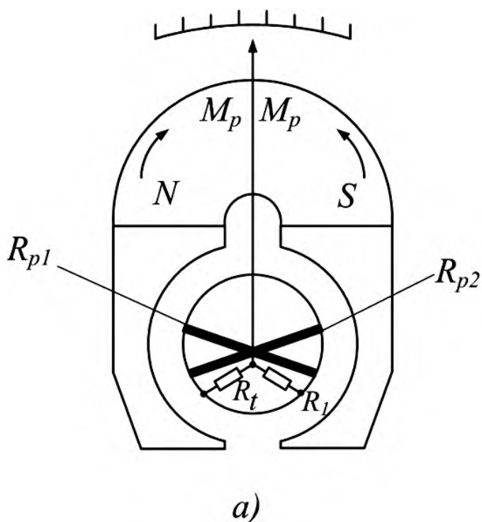
Рис. 3.3. Устройство магнитоэлектрического логометра (a) и его измерительная схема (б)
