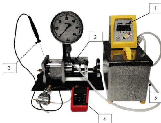
Рисунок 7.5 – Конструкция изделия: 1 – навесной термостат; 2 – прибор для определения критической температуры; 3 – термопара; 4 – цифровой быстродействующий карманный термометр; 5 – силиконовая трубка;
