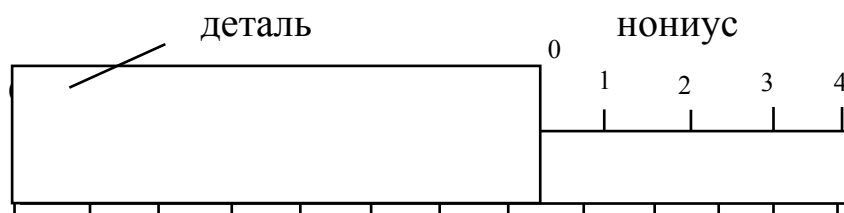
Рисунок 2.1 – Нониус и основная шкала
