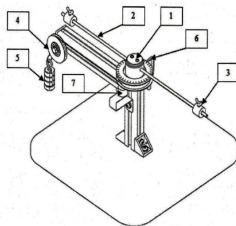
Рисунок 2.3 – Конструкция изделия:
