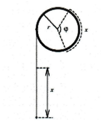
Рисунок 2.1 – Схема блока с натянутой капроновой нитью
