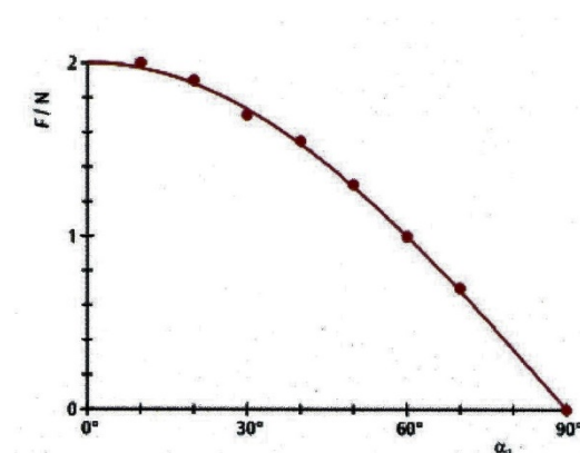
Рисунок 4.4 – Измеренная и рассчитанная суммы двух симметричных сил в зависимости от угла a_1
