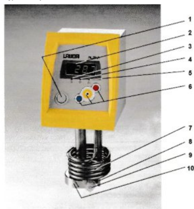
Рисунок 7.7 – навесной термостат Alpha: 1 – сетевой выключатель; 2 – регулятор температуры с четырех разрядным светодиодным указателем; 3 – нагревательное устройство активно (горит желтый светодиод); 4 – устройство охлаждения активно (горит синий светодиод); 5 – сигнал неисправности (мигает красный светодиод); 6 – функции меню, клавиша выбора и ввода; 7 – нагревательный элемент; 8 – датчик температуры Pt100; 9 – отвод насоса с дросселем расхода; 10 – корпус насоса;
