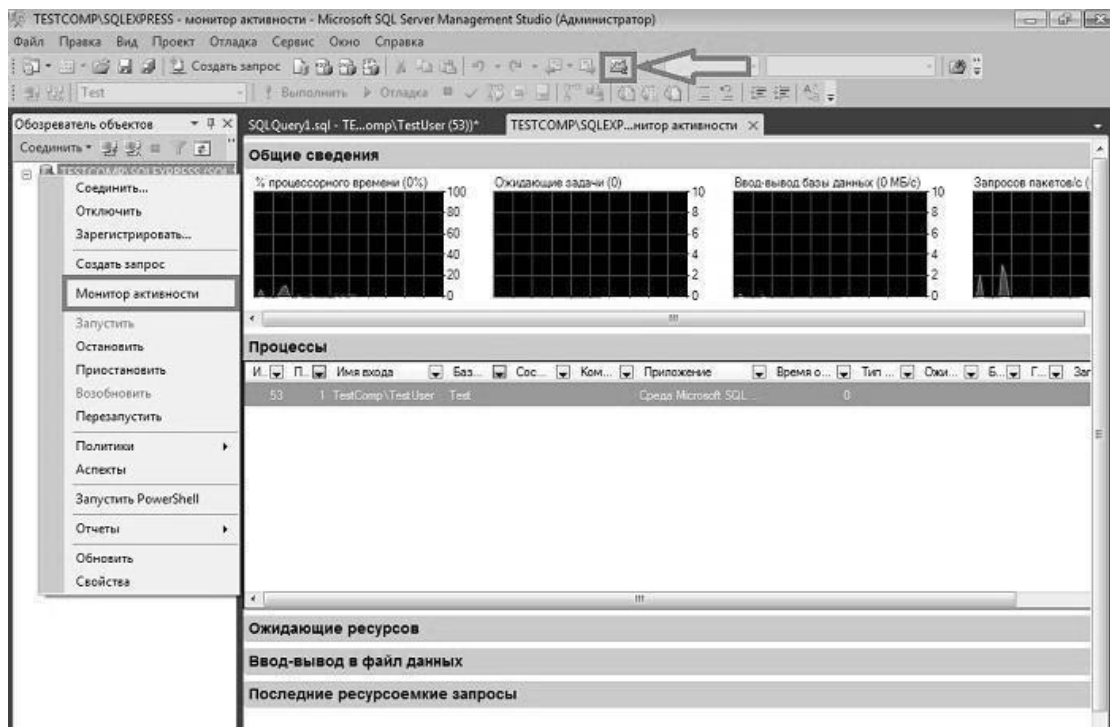
Рис. 5.8. Монитор активности
