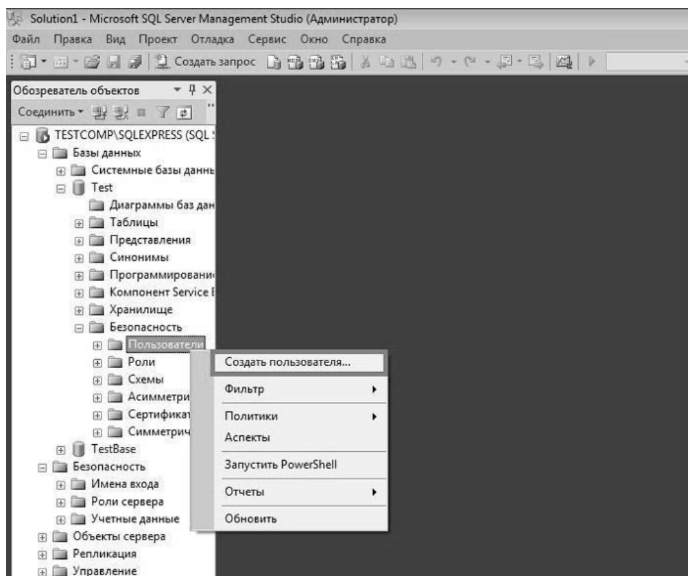
Рис. 5.13. Создание пользователя
