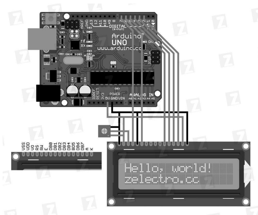
Рис. 4.2. Прямое подключение к Arduino
