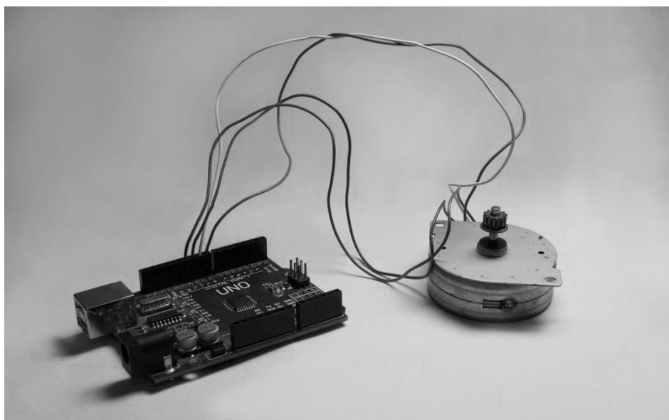
Рис. 3.2. Соединенные плата Arduino и ШД
