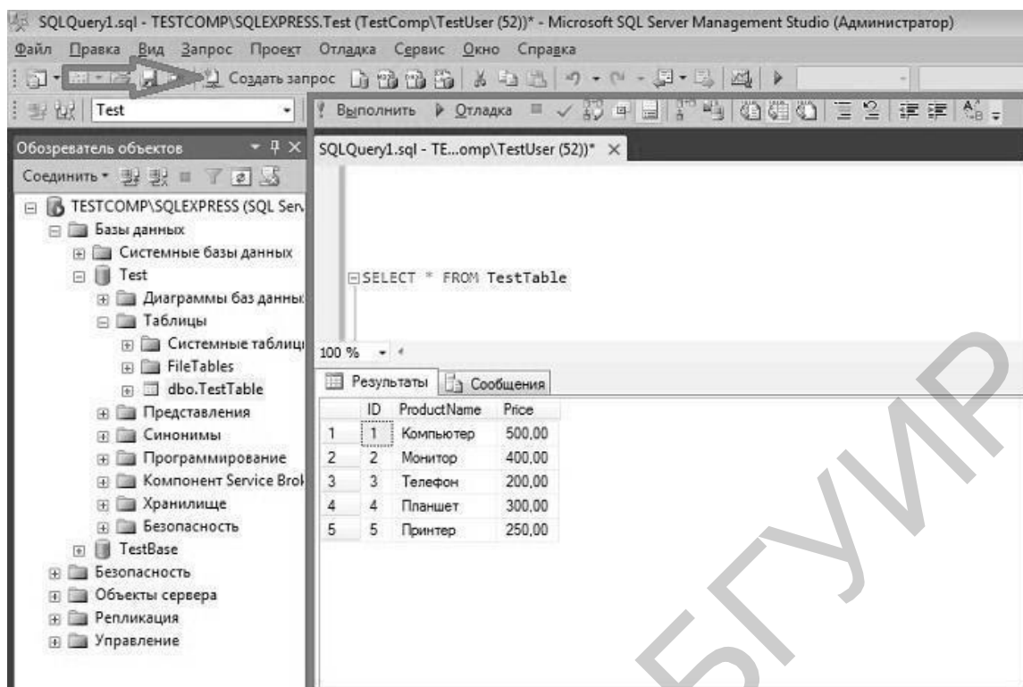
Рис. 5.4. Создание и редактирование сценариев
