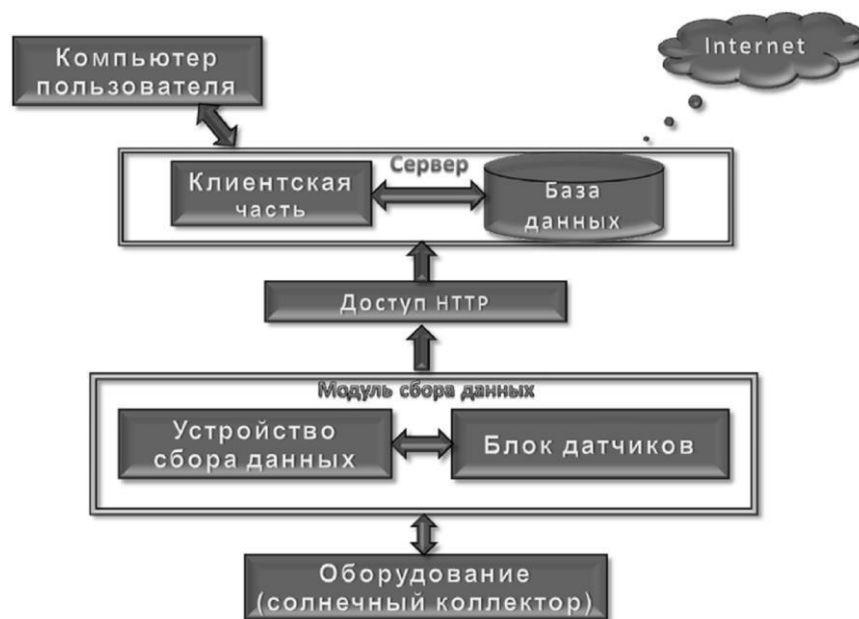
Рис. 5.1. Структурная схема системы сбора и обработки результатов измерений и мониторинга
