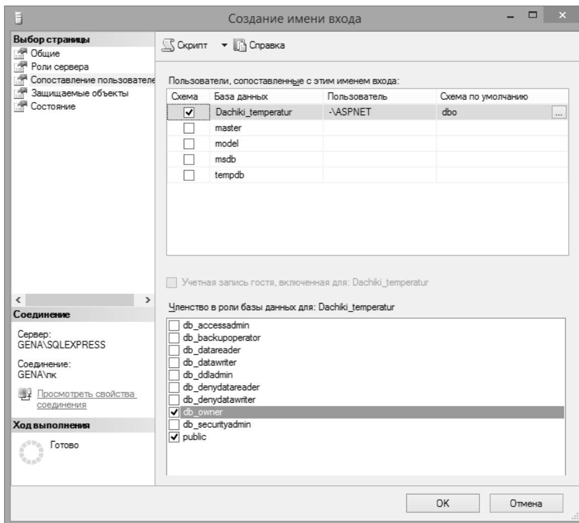
Рис. 6.8. Настройка свойств учетной записи ASP.NET (выбор ролевого членства для базы данных)
