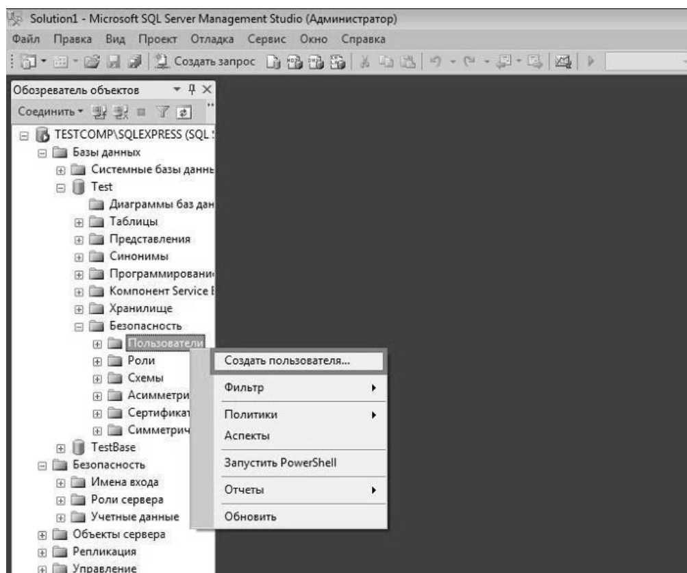
Рис. 5.13. Создание пользователя
