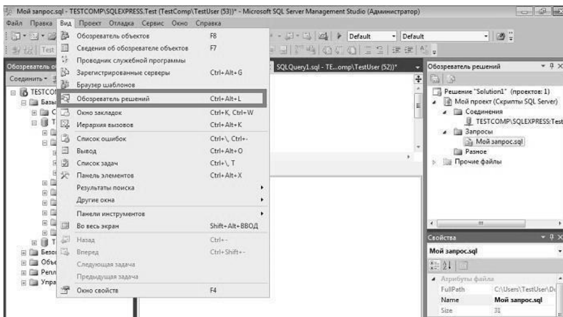
Рис. 5.6. Обзорщик решений
