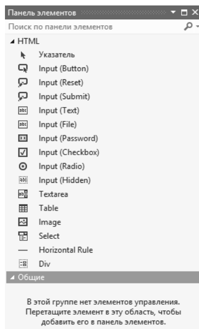
Рис. 6.4. Панель элементов
