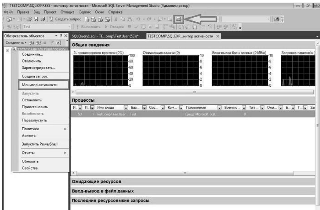
Рис. 5.8. Монитор активности
