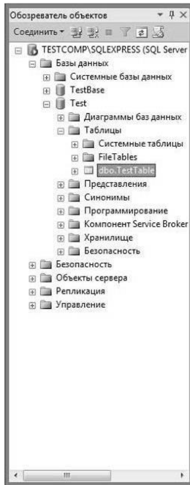
Рис. 5.3. Обзорщик объектов
