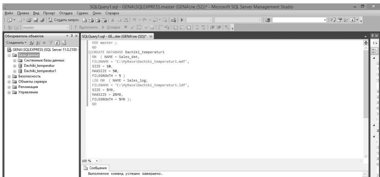
Рис. 5.19. Создание новой базы программным путем
