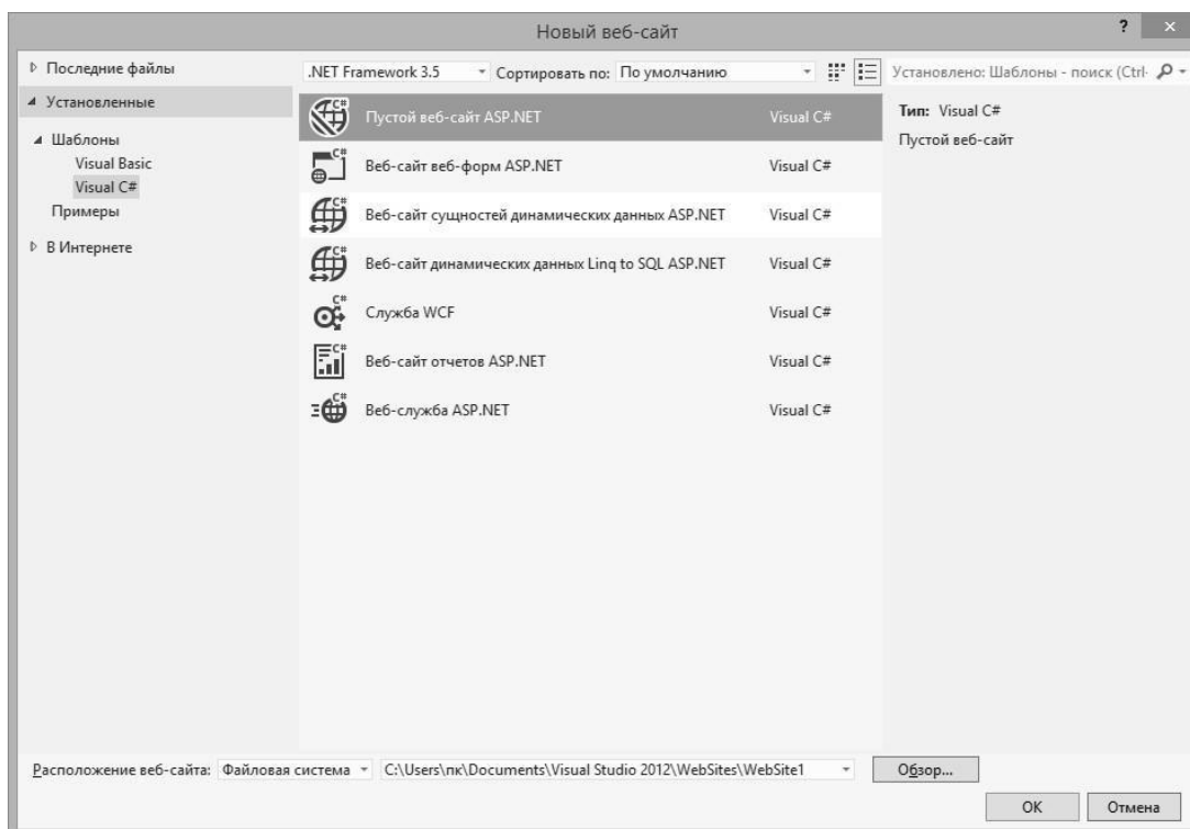
Рис. 6.2. Формирование шаблона
