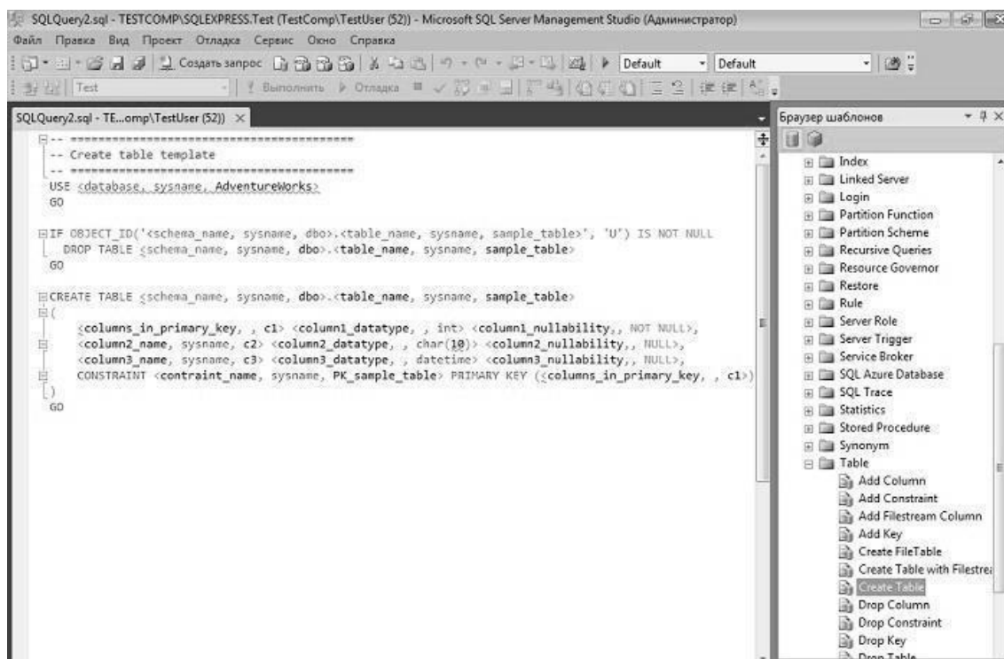
Рис. 5.7. Браузер шаблонов
