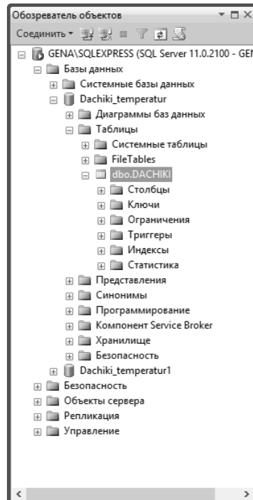
Рис. 5.21. Созданная таблица
