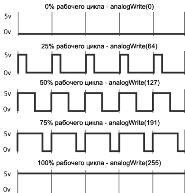
Рис. 2.1. Широтно-импульсная модуляция
