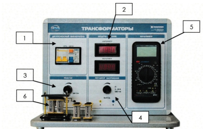
Рисунок 12.3 – Конструкция изделия
