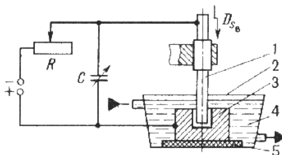
Рисунок 8.7 – Схема электроискрового станка: 1 – электрод-инструмент; 2 – ванна; 3 – заготовка-электрод; 4 – диэлектрическая жидкость; 5 – изолятор
