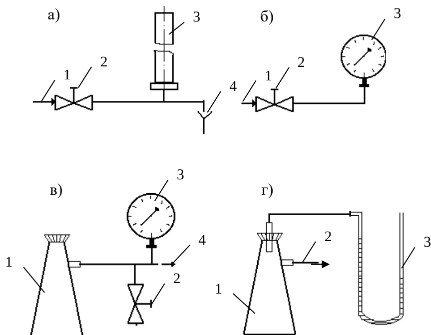
Рис. 4. Схемы экспериментальных установок для измерения давления:
