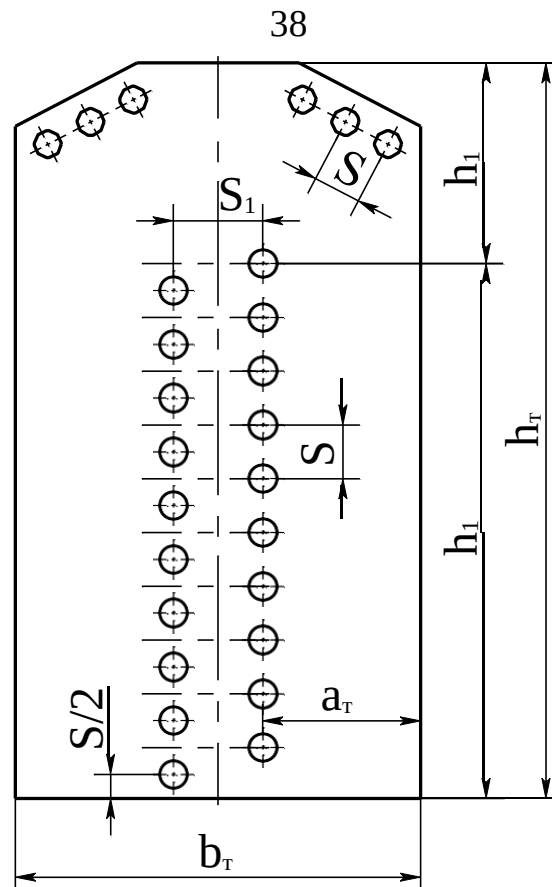
Рисунок 3.3 – Схема к определению размеров камеры радиации
