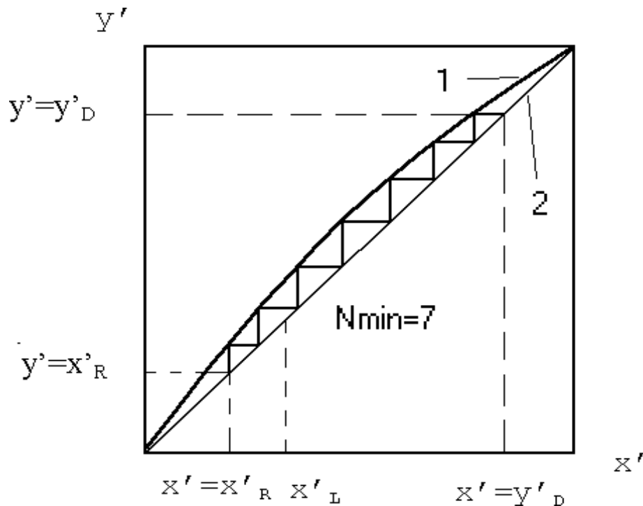
Рис. 2. Определение числа ступеней контактирования по диаграмме y'-x' : 1 - линия равновесия; 2 - рабочая линия (при \gamma \rightarrow \infty ).
