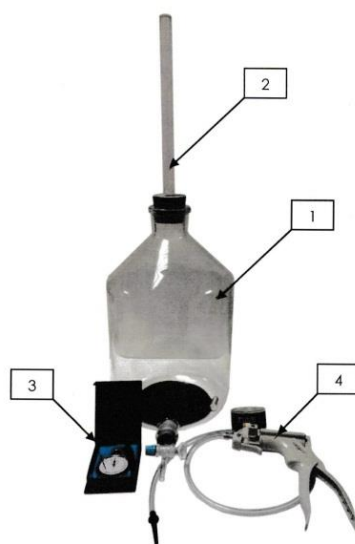
Рисунок 8.2 – Конструкция изделия: 1 – Бутылка Мариотта; 2 – колебательная трубка; 3 – механический секундомер; 4 – ручной вакуумный насос;
