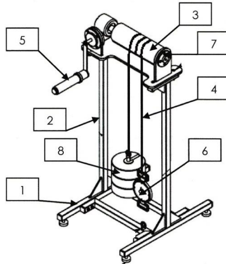
Рисунок 6.1 – Конструкция изделия
