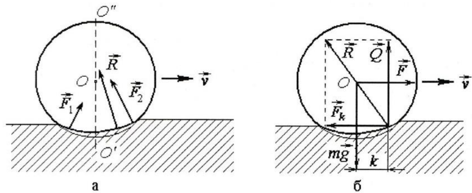
Рисунок 5.2 – а) Возникновение силы в случае неупругой деформации катящегося тела и поверхности; б) движение цилиндрического тела массой m по горизонтальной поверхности под действием внешней силы \bar{F} .
