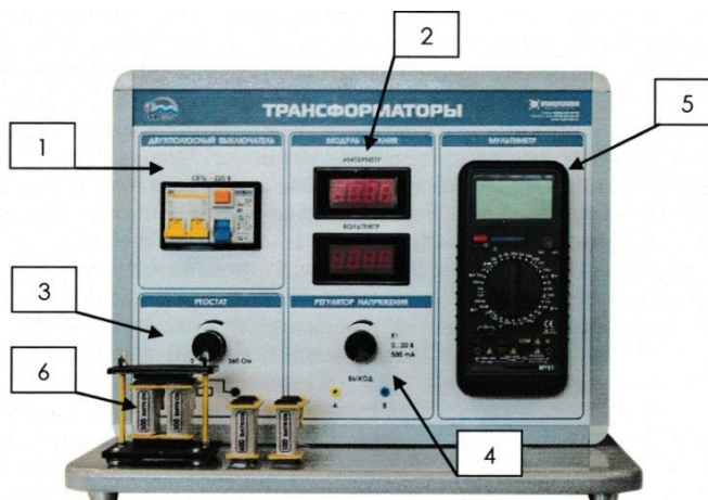
Рисунок 10.1 – Конструкция изделия
