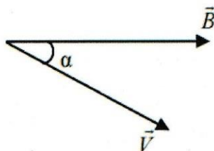
Рисунок 16.2 – К расчету модуля силы Лоренца
