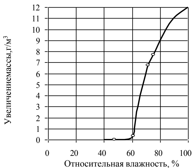
Рисунок 1.2 – Коррозия железа в воздухе, содержащем 0,01 % (об.) SO_2
