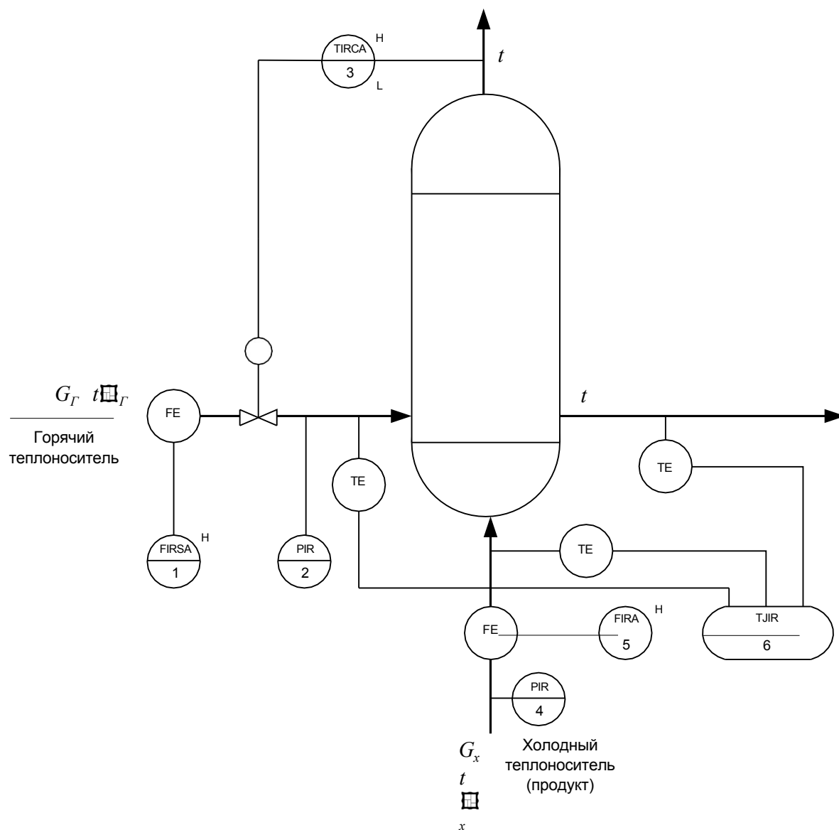
Рисунок 2 – Схема автоматизации (упрощенная) кожухотрубного теплообменника
