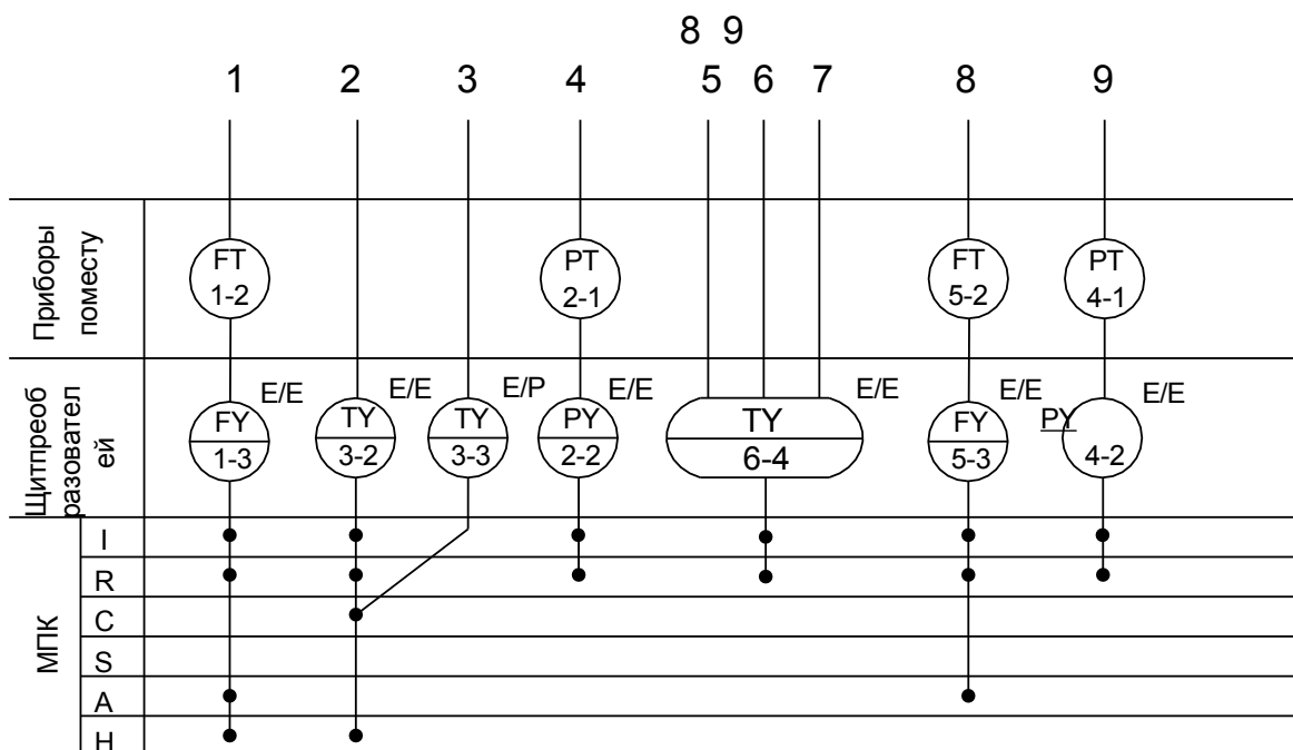
Рисунок 3 – Схема автоматизации (развернутая) кожухотрубного теплообменника
