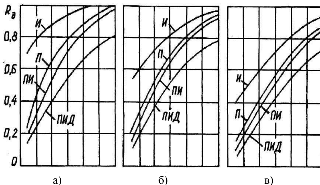
Рисунок 2 – Динамические коэффициенты регулирования на статических объектах: а – апериодический процесс; б – процесс с 20%-ным перерегулированием; в – процесс с \min \int_0^\infty X_{\text{вых}}^2(t)dt ,
