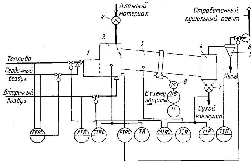
Рисунок А.14 – Схема автоматизации процесса сушки:
