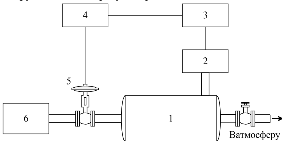
Рисунок 4.3 – Конструктивно-функциональная схема АСР,
