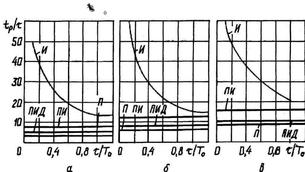
Рисунок 3 – Время регулирования на статических объектах: а –
