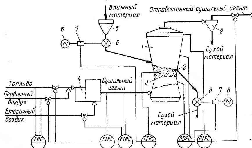
Рисунок А.16 – Схема автоматизации процесса сушки в сушилках с кипящим слоем:
