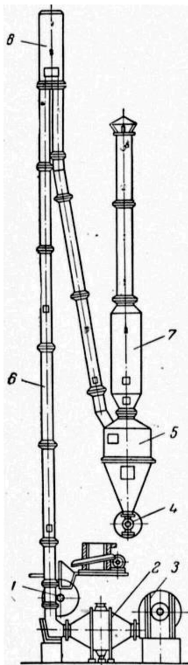
Рисунок 3.5 – Пневматическая труба-сушилка
