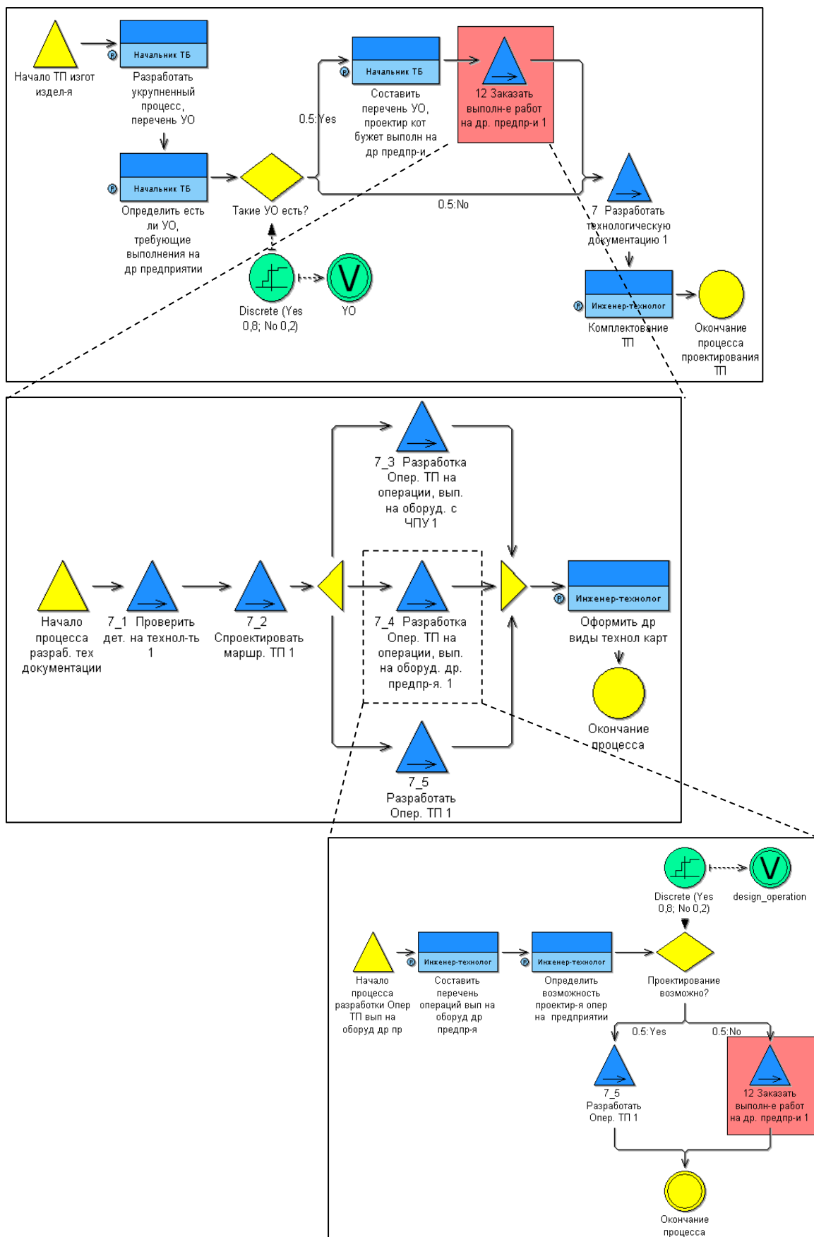
Рис. 22. Модель «Разработка технологического процесса», выполненная в системе Adonis
