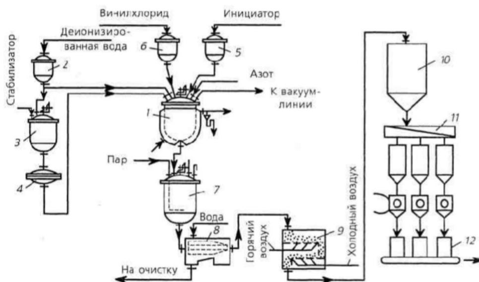
Рис. 8.2. Схема производства поливинилхлорида и суспензии: 1 — реактор; 2 — емкость деионизированной воды; 3 — емкость раствора стабилизатора; 4 — фильтр; 5 — весовой мерник раствора инициатора; 6 — сборник поливинилхлорида; 7 — сборник-усреднитель; 8 — центрифуга; 9 — сушилка; 10 — бункер; 11 — узел рассева порошка; 12 — тара для порошка поливинилхлорида
