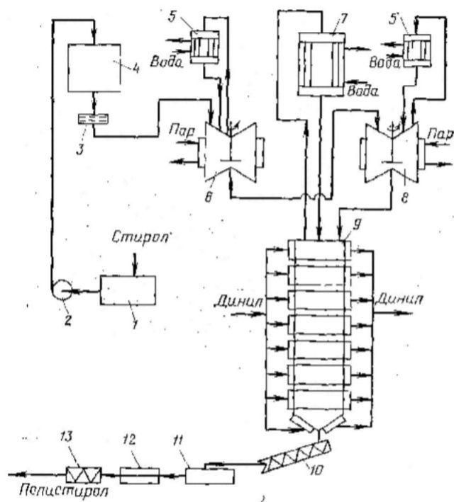
Рисунок 1. Технологическая схема процесса получения блочного полистирола:
