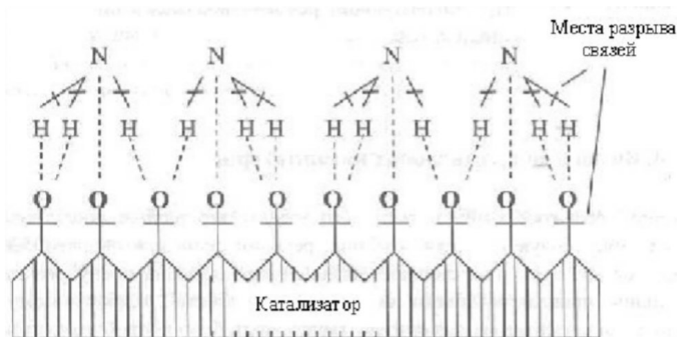
Рис. 2.33. Мысленная схема окисления аммиака на поверхности платинового катализатора (сплошными линиями обозначены химические связи в молекулах реагентов адсорбционные связи, пунктирными - образованные связи вследствие катализа)
