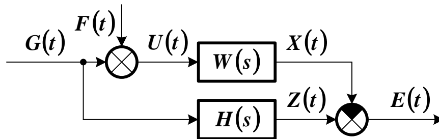
Рисунок 3.3 – Схема преобразования полезного сигнала
