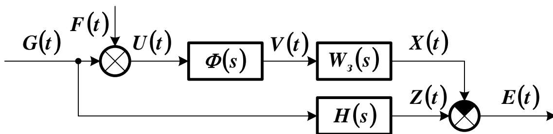
Рисунок 3.4 – Схема преобразования полезного сигнала с использованием отбеливающего фильтра
