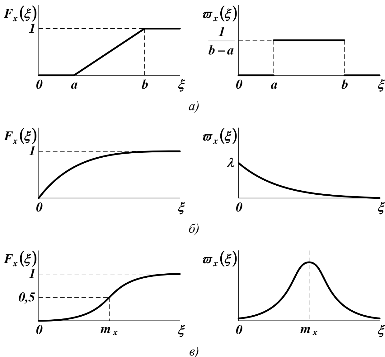
Рисунок 1.2 – Функции распределения и плотности вероятности: (а) равномерное распределение; (б) экспоненциальное распределение; (в) нормальное распределение
