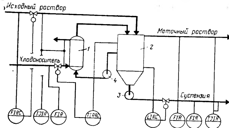
Рисунок А.12 – Схема автоматизации процесса кристаллизации:
