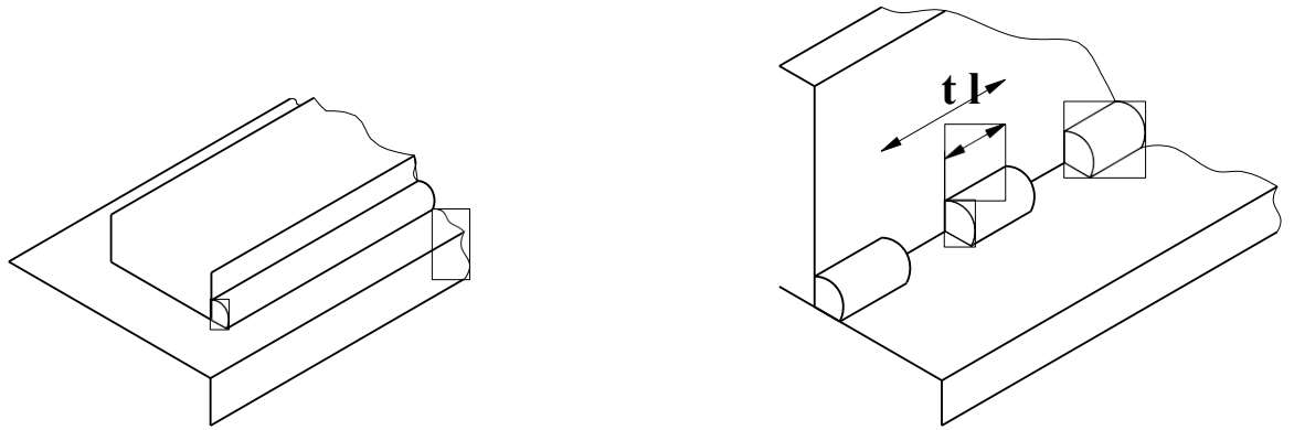
Рисунок 3.33 - Швы сплошные (а) и прерывистые (б)
