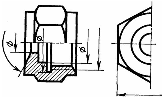
Рисунок 4.25 – Простановка размеров при соединении вида и разреза
