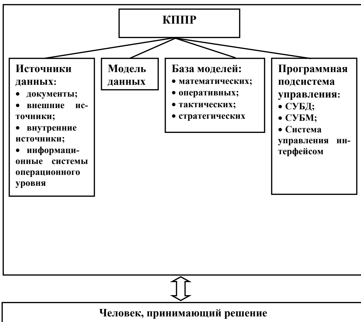
Рис. 2. Структура КППР
