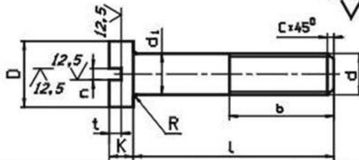
Винты с цилиндрической головкой класса точности В (нормальной точности) ГОСТ 1491-50
