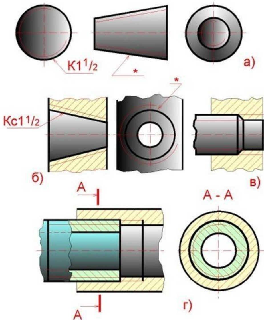
Рисунок 20.7 – Изображение резьб
