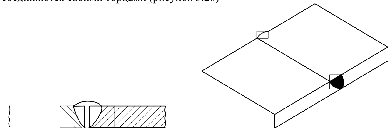
Рисунок 3.28 – Стыковые швы
