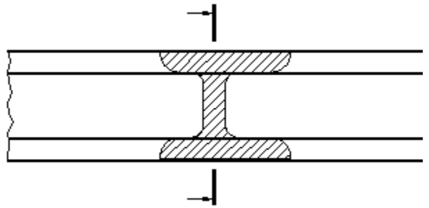
Рисунок 2.25 – Обозначение несимметричного наложенного сечения.
