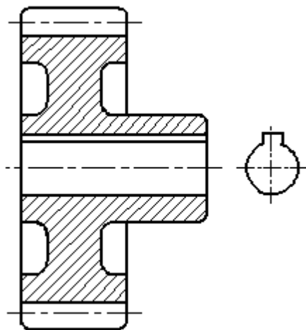
Рисунок 2.49 – Образец изображения отверстия в ступице зубчатого ко- леса.
