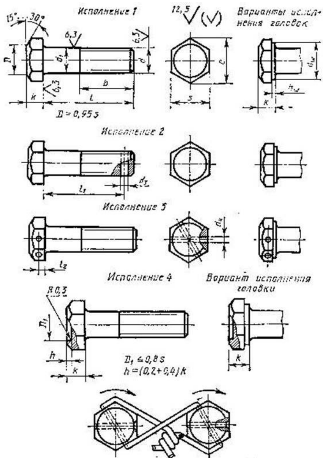
Рисунок 3.12 – Изображение болта
