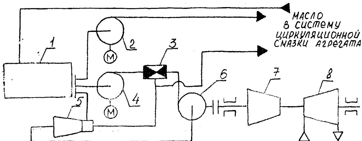
Схема технологического объекта управления
