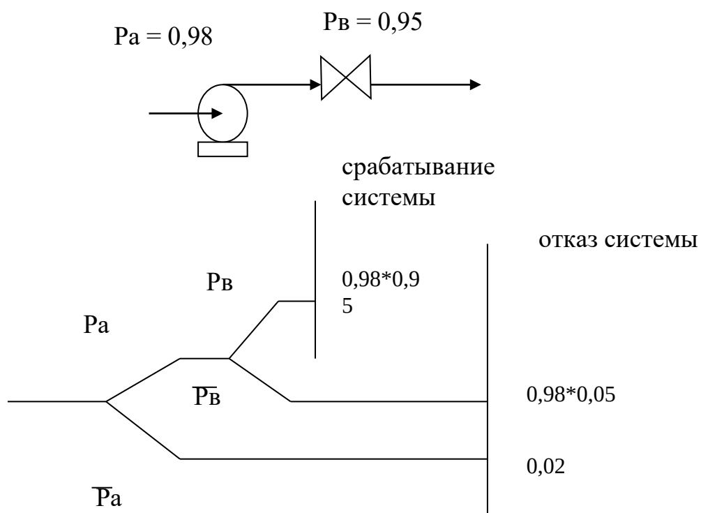
Рисунок 2.1 – Расчетная схема
