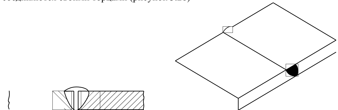
Рисунок 3.28 – Стыковые швы
