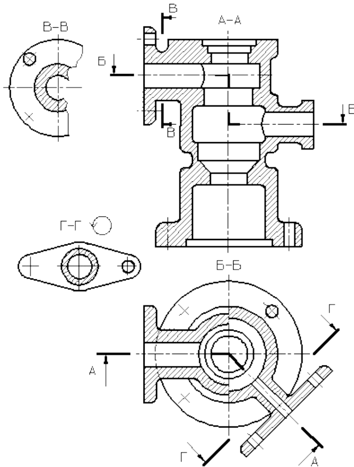
Рисунок 2.7 – Виды разрезов.
