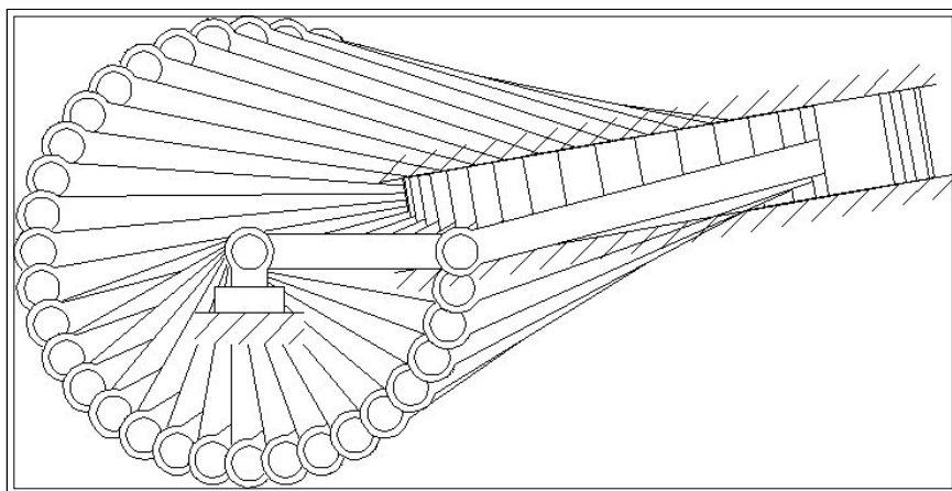
Рисунок 86 – Анимация механизма
