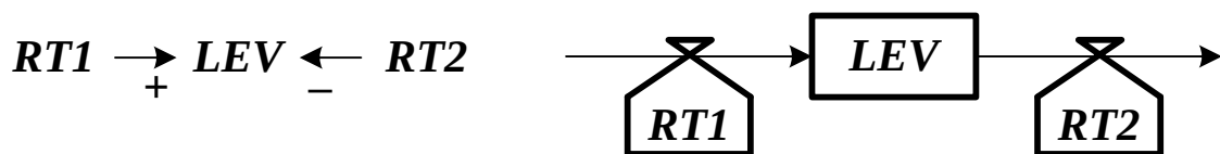
Рисунок 1.4 — Диаграмма причинно-следственных связей и диаграмма потоков и уровней для однопоточной системы
