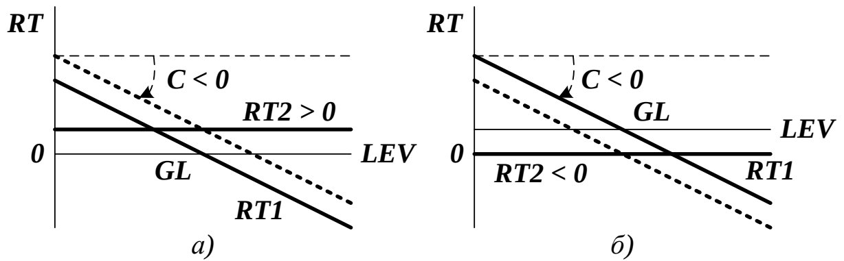
Рисунок 1.2 — Нагрузочная характеристика системы (а) с положительным и (б) отрицательным возмущением
