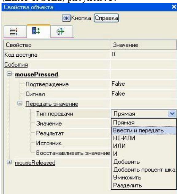
Рисунок 95 – Настройка типа передачи
