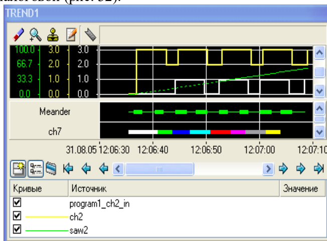
Рис. 32. ГЭ Тренд
