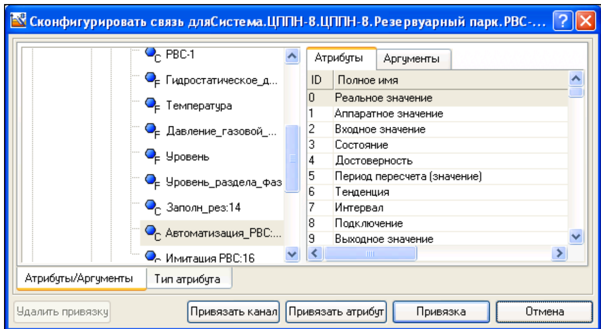
Рис. 55. Диалоговое окно конфигурирования привязки
