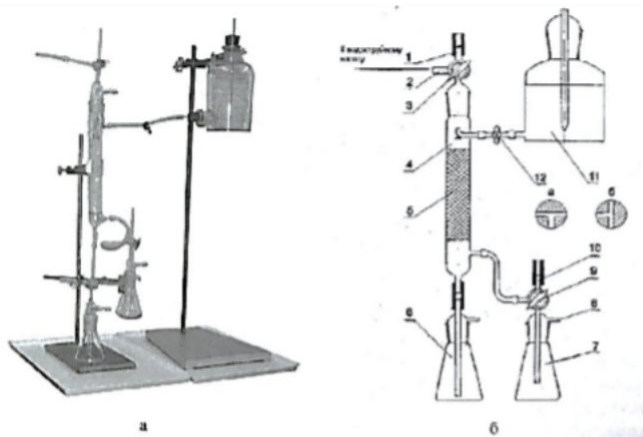
Рисунок 30. Абсорбционная установка:
