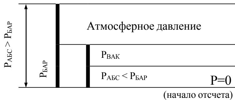
Рис. 1 Взаимосвязь P_{\text{ABS}} ; P_{\text{BAP}} ; P_{\text{ИЗБ}} и P_{\text{ВАК}} .
