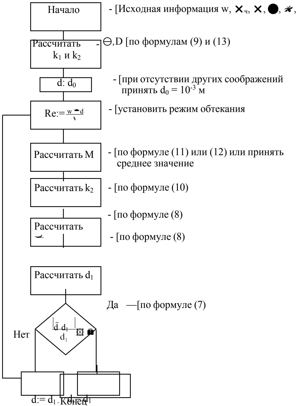
Рис. 4. Схема алгоритма вычисления диаметра фракции.
