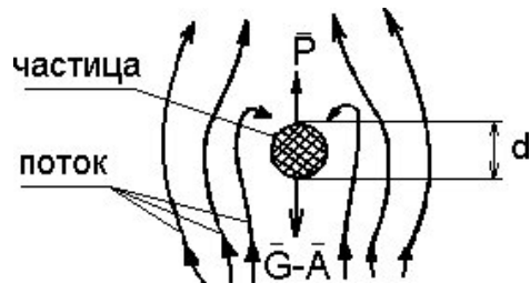
Рис. 1. Схема сил, действующих на частицу в потоке среды.
