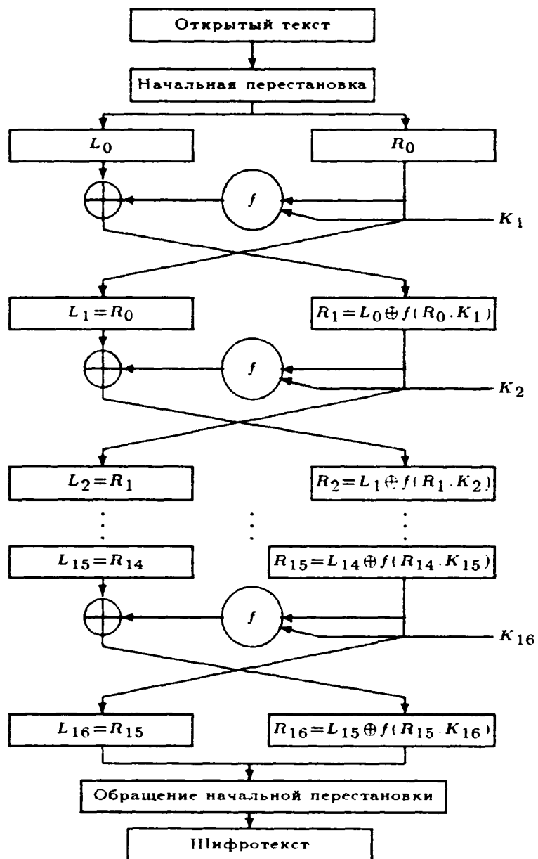
Рисунок 3.6 – Схема DES-преобразования
