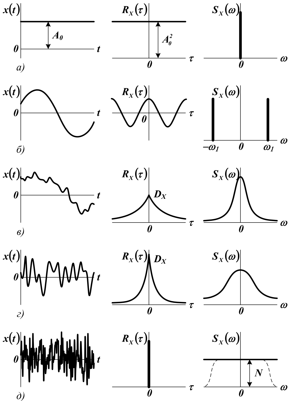
Рисунок 1.5 – Корреляционные функции и спектральные плотности случайных процессов различной структуры
