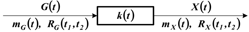
Рисунок 2.1 – Линейная система с весовой функцией k(t) , находящаяся под влиянием случайного воздействия
