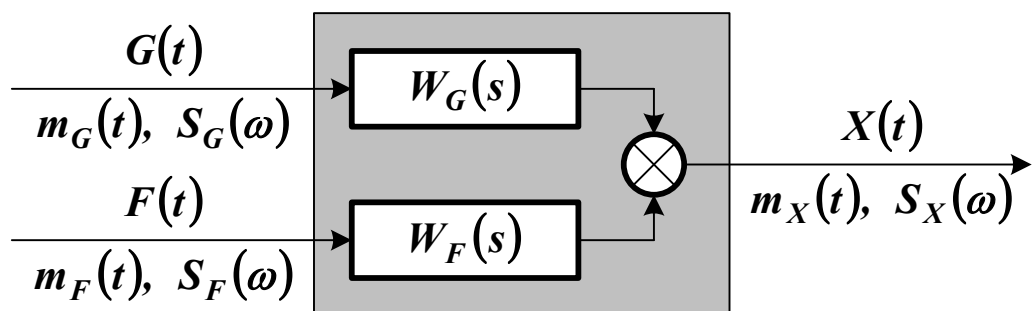
Рисунок 2.5 – Система, находящаяся под влиянием двух случайных воздействий
