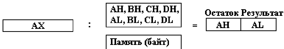
Рисунок 1.6 – Возможные способы размещения делимого, делителя и результата: а – операнды-слова, б – операнды-байты
