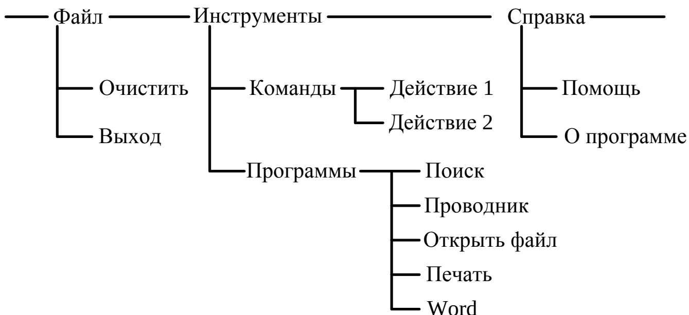
Рисунок 4 – Структура меню задания на лабораторную работу
