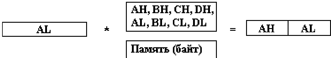
Рисунок 1.5 – Возможные способы размещения сомножителей и результата: а – операнды-слова, б – операнды-байты
