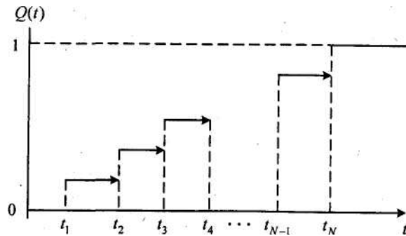
Рис. 1.3. График статистической вероятности отказа элемента
