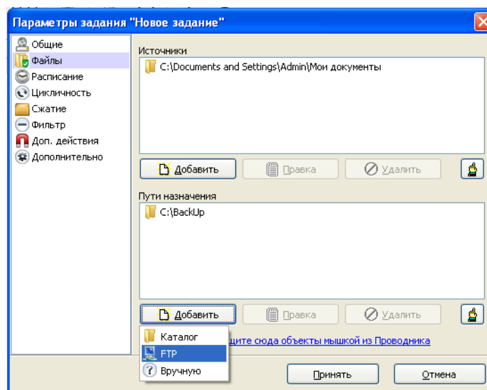
Рисунок 9. Окно параметров Нового задания Cobian Backup. Вкладка Файлы .
