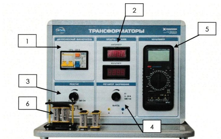
Рисунок 10.1 – Конструкция изделия
