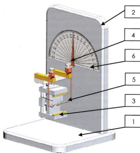
Рисунок 16.4 – Конструкция изделия
