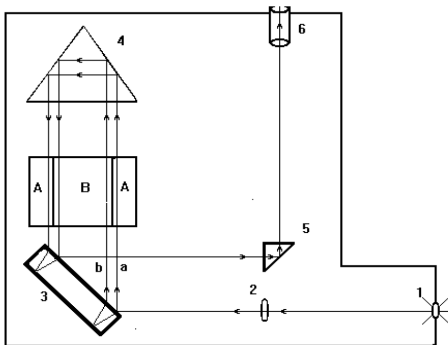
Рисунок 19.2 – Рабочая схема интерферометра ШИ-5
