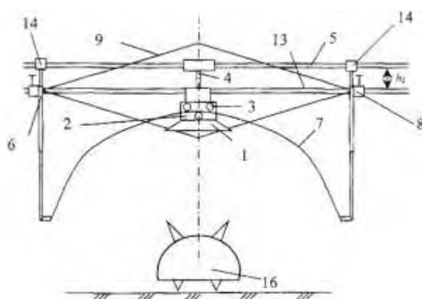
Фигура 4 – Вариант облучателя
