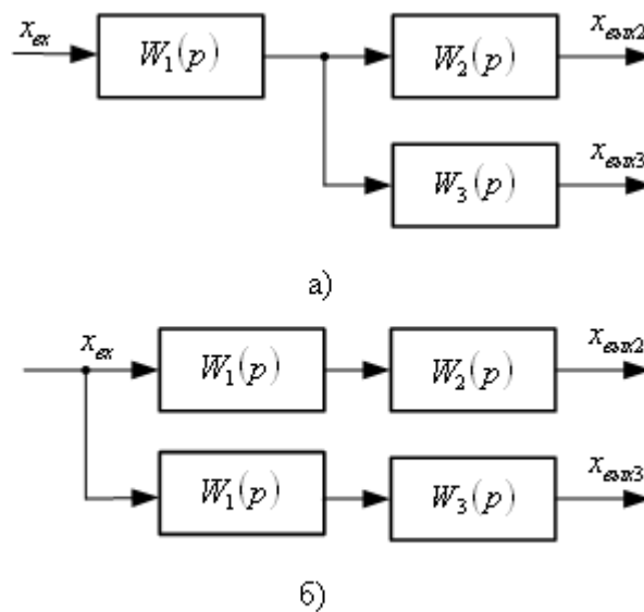
Рисунок 6 – Эквивалентное преобразование: а) исходная схема; б) схема, полученная в результате переноса воздействия f на выход звена 6. Точку присоединения любой структурной связи к выходу звена, имеющего передаточную функцию W_1(p) , можно перенести на его вход, включив в эту связь дополнительное звено с той же передаточной функцией W_1(p) :
