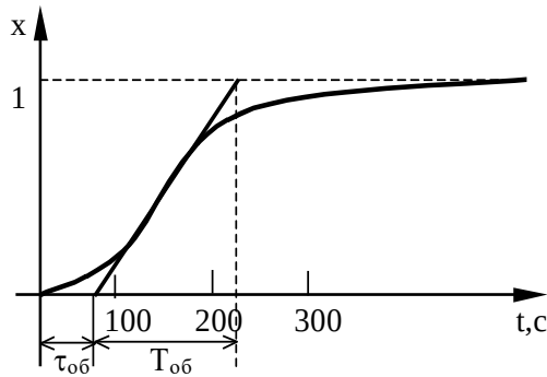
Рисунок 1 – Оценка параметров \tau_{об} , T_{об} , K_{об.p} по кривой разгона объекта регулирования
