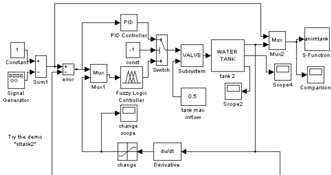
Рис. 2. Блок-диаграмма модели системы управления уровнем воды в баке нечётким регулятором
