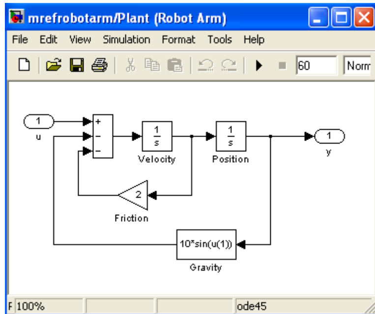
Рис. 14. Структурная динамическая модель звена робота
