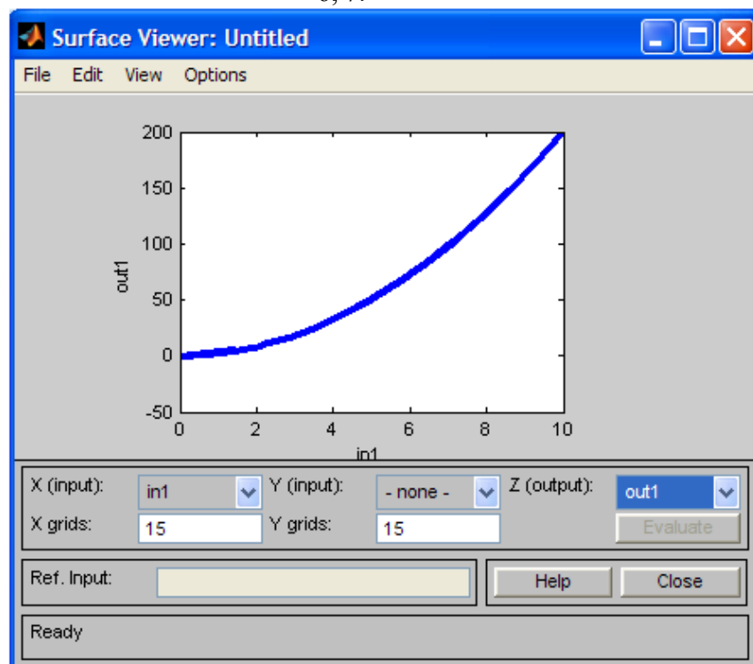
Рис.6. Поверхность системы нечеткого вывода
