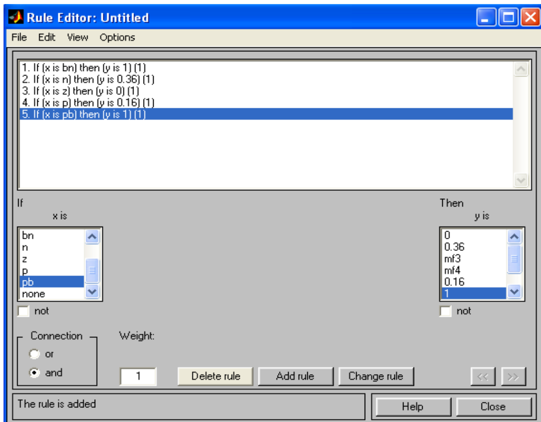
Рис. 2.5. Окно редактора правил
