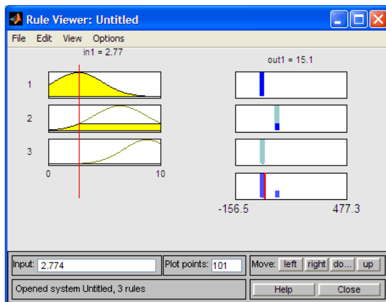
Рис.7. Нечеткие правила, полученные при обучении Индивидуальное задание
