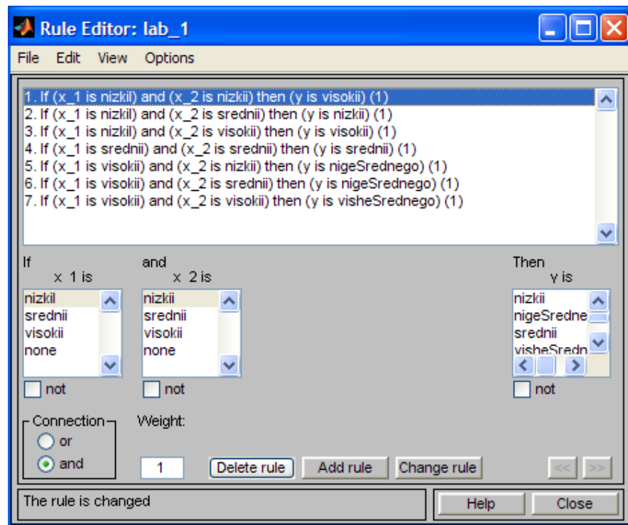
Рис. 4. Нечеткая база знаний Mamdani
