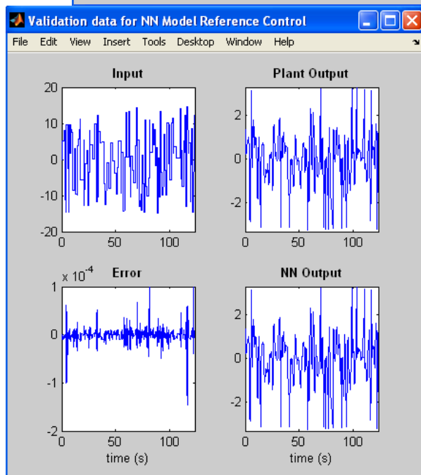
Рис. 20. Результат обучения модели на обучающем множестве
