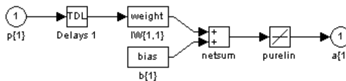
Рис. 8. Структура созданной НС
