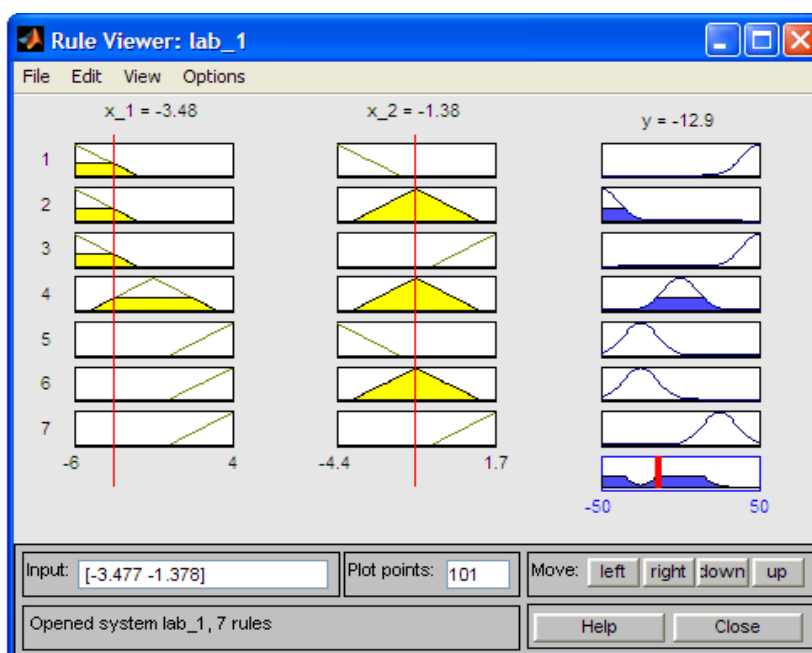
Рис. 5. Визуализация нечеткого вывода Mamdani
