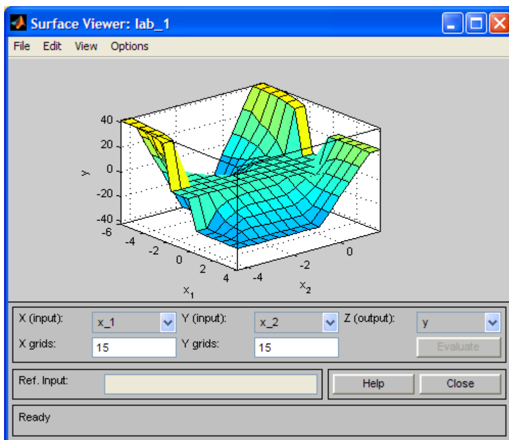
Рис. 6. Поверхность «входы выход» для базы знаний в Surface Viewer
