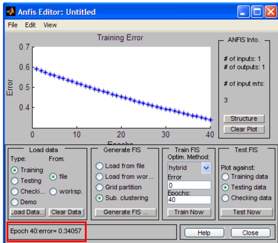
Рис. 5. Процесс обучения нейронной сети
