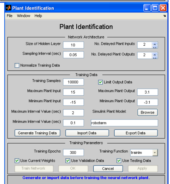
Рис. 17. Окно для построения нейросетевой модели ОУ
