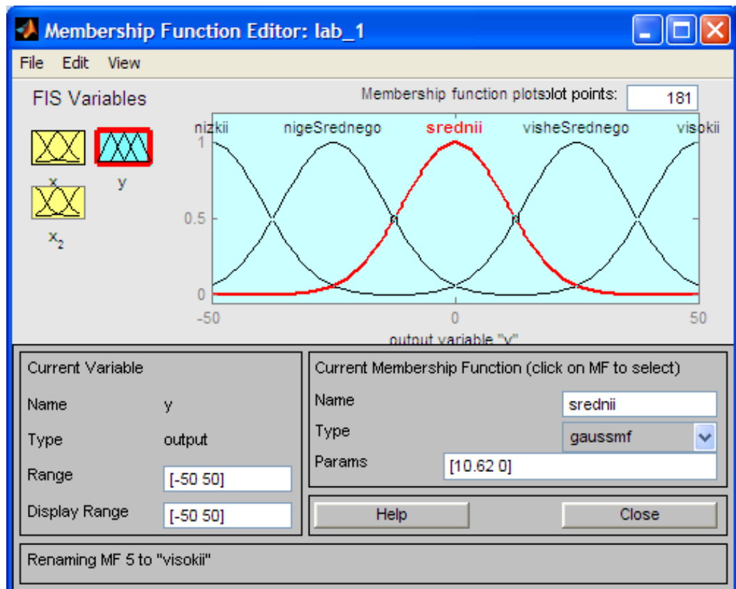
Рис.3. Функции принадлежности переменной y
