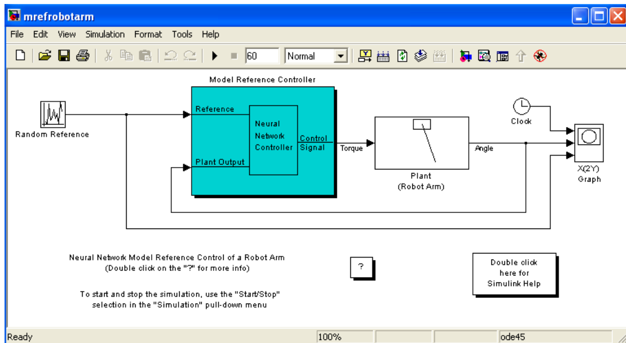
Рис. 12. Структура нейросетевой системы управления в среде Simulink
