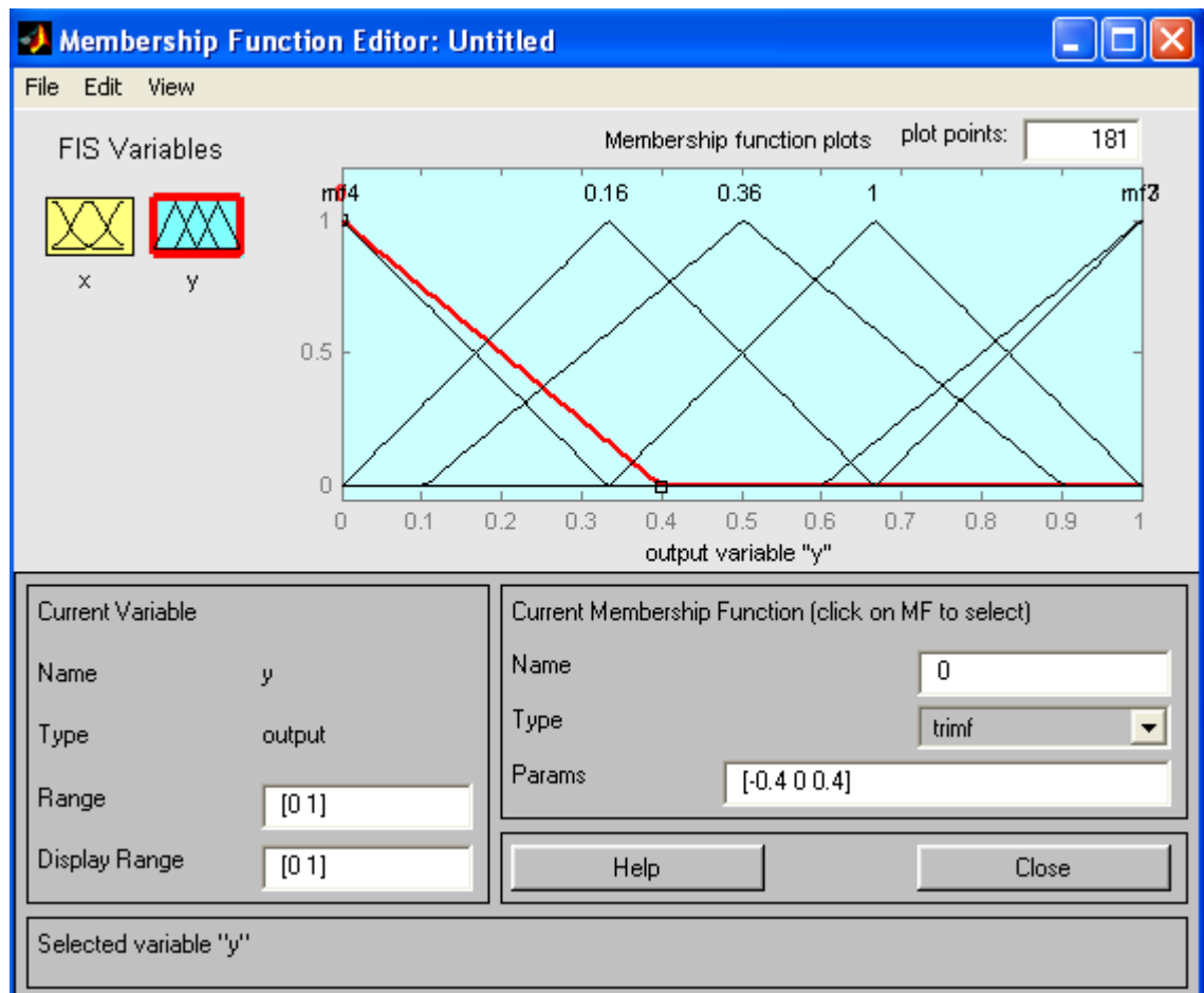
Рис. 2.4. Параметры функций принадлежности переменной y
