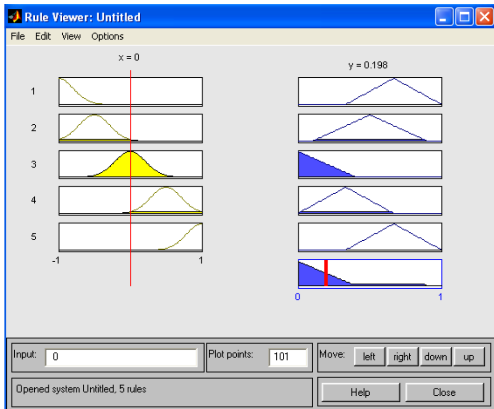
Рис. 2.6. Окно просмотра правил
